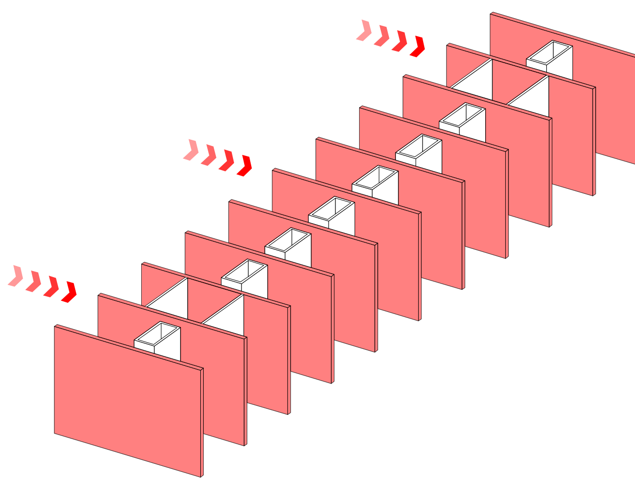
Aussteifung Windlast Querrichtung
