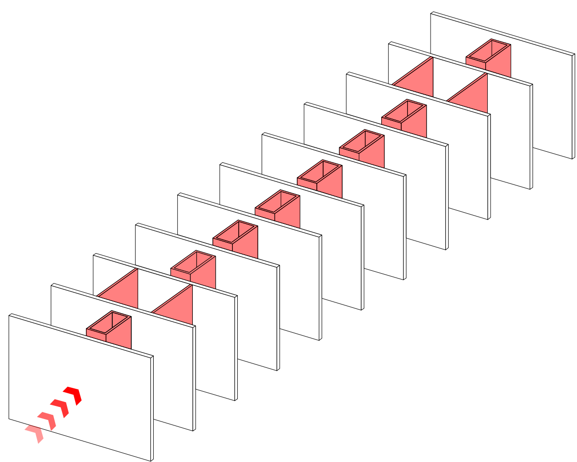
Aussteifung Windlast Längsrichtung
