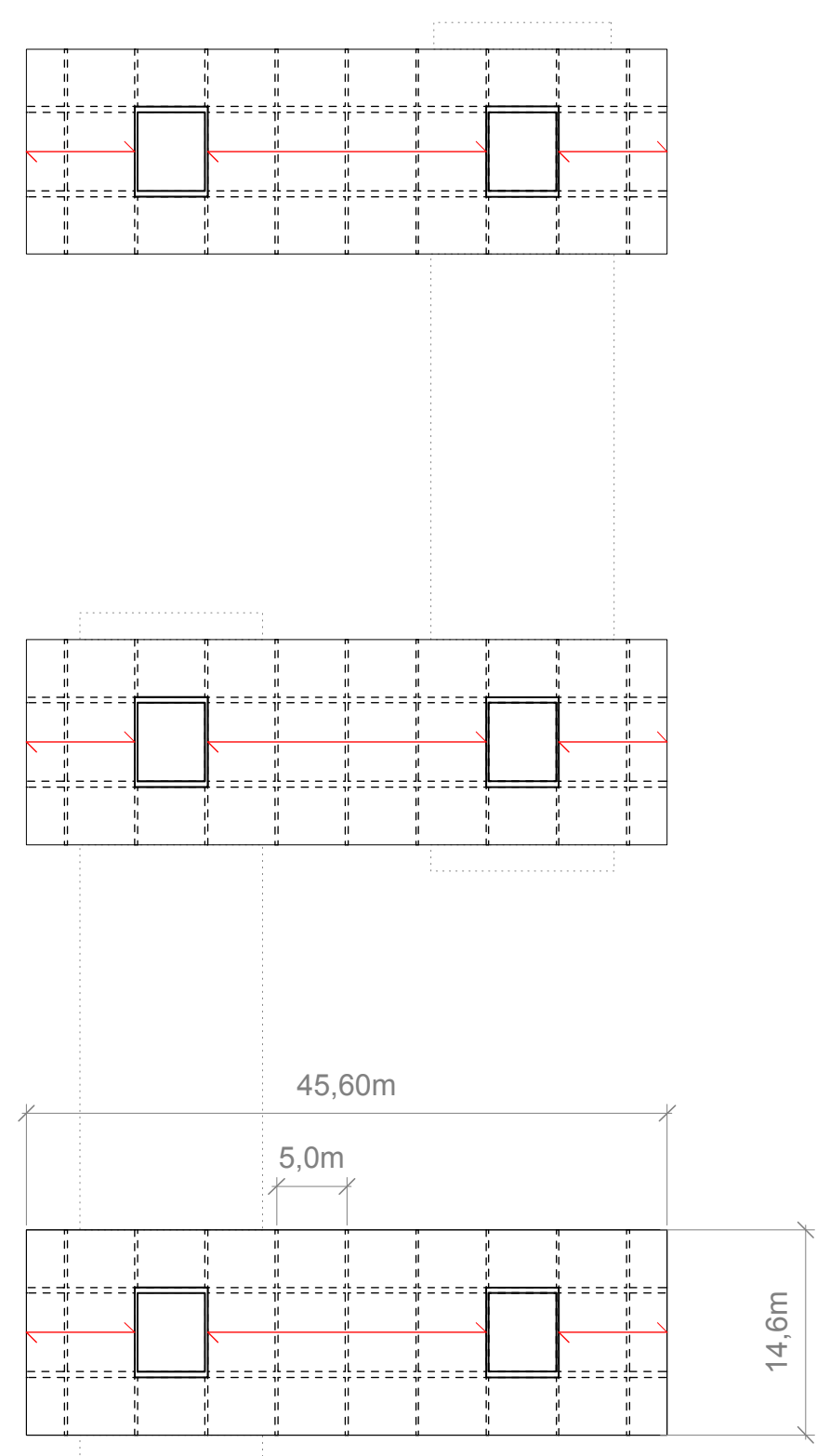
3.OG,4.OG,5.OG Deckenspannrichtung 1:500
