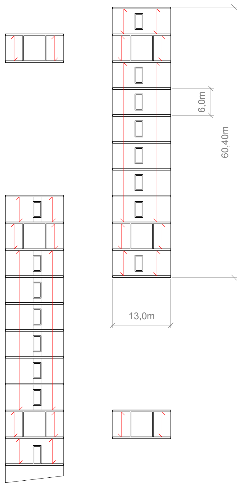
EG,1.OG,2.OG Deckenspannrichtung 1:500
