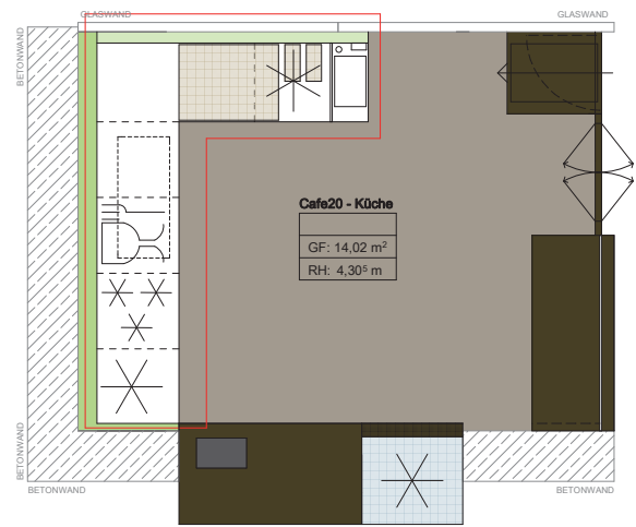
Übersichtsplan M 1:50
