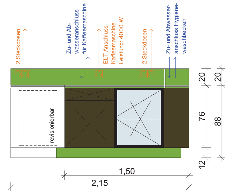
Ansicht (kurze Seite) M 1:20
