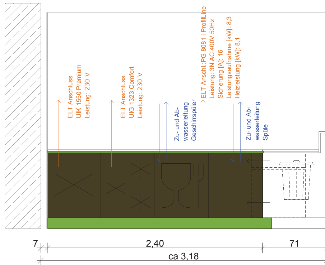
Ansicht (lange Seite) M 1:20
