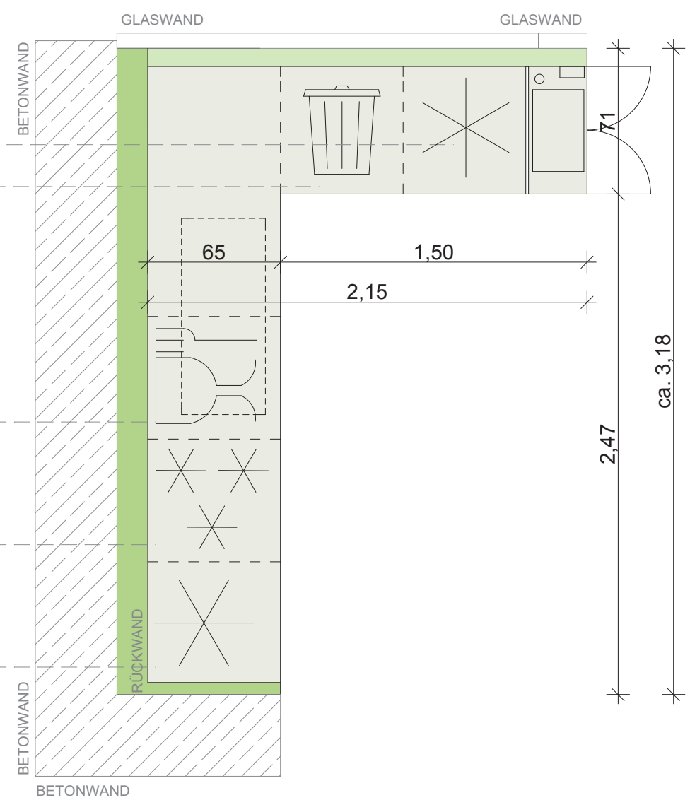
Grundriss M 1:20
