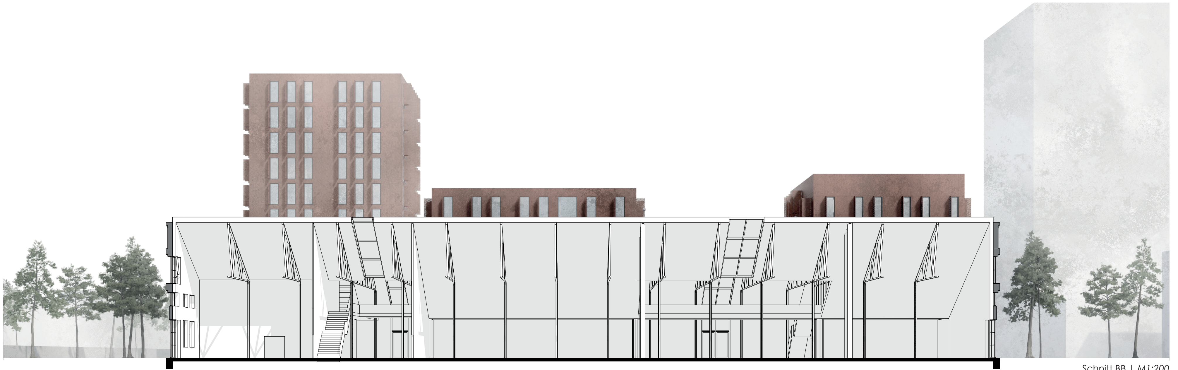
Schnitt BB | M1:200
