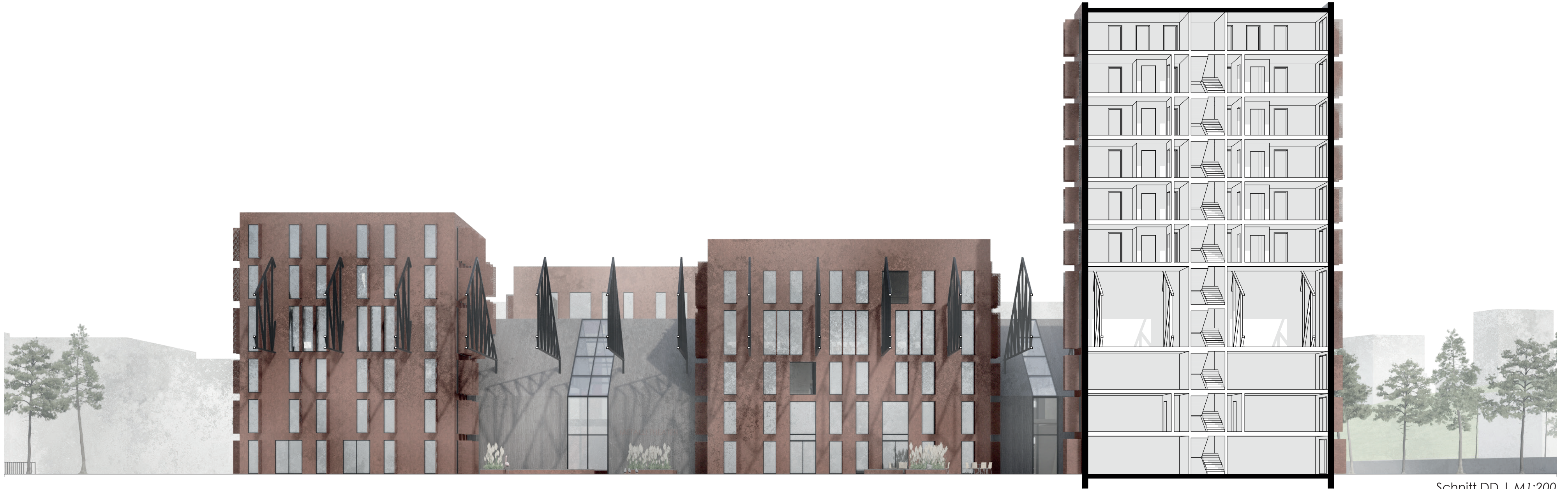
Schnitt DD | M1:200
