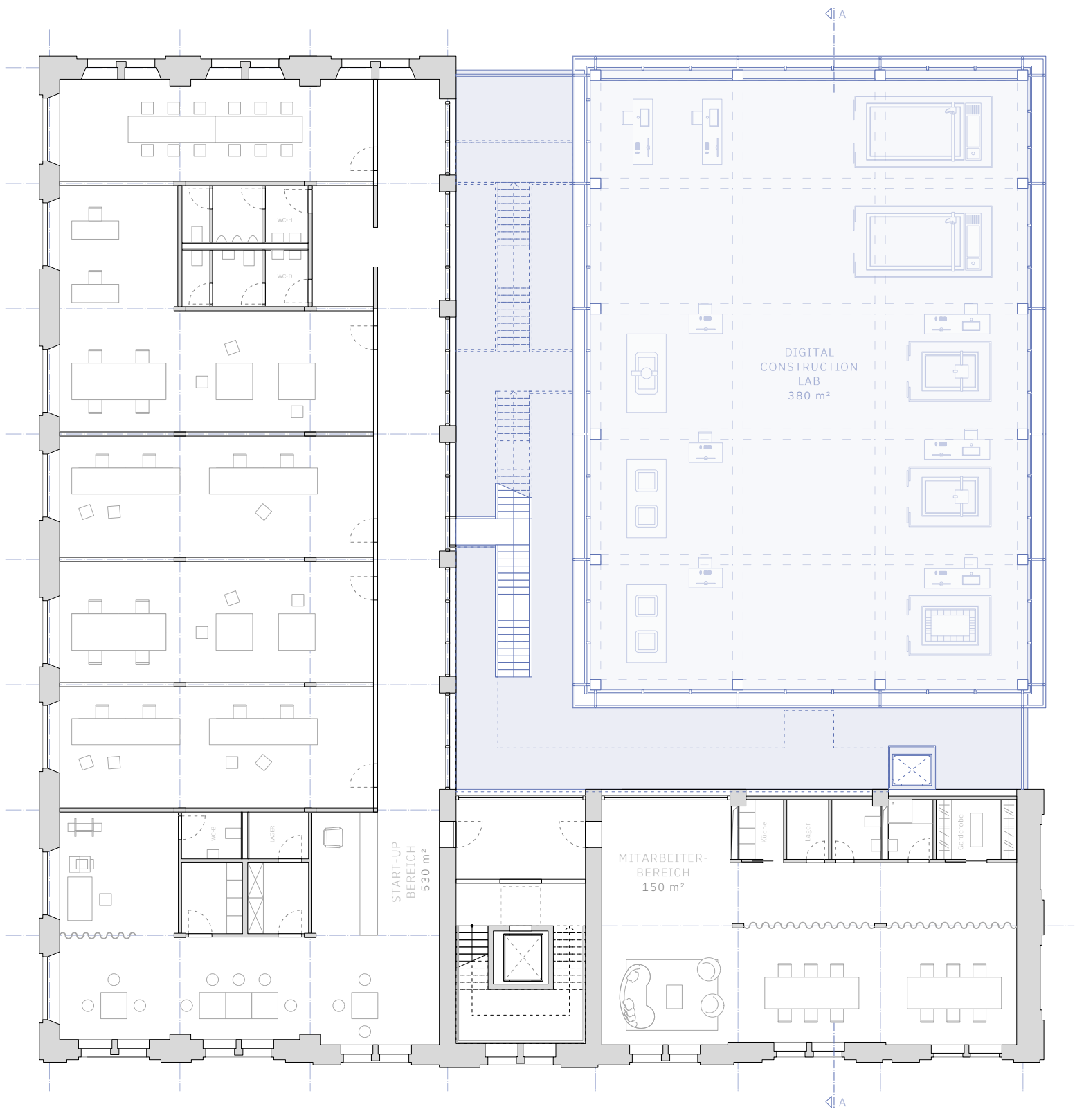
GRUNDRISS - 1. OBERGESCHOSS
