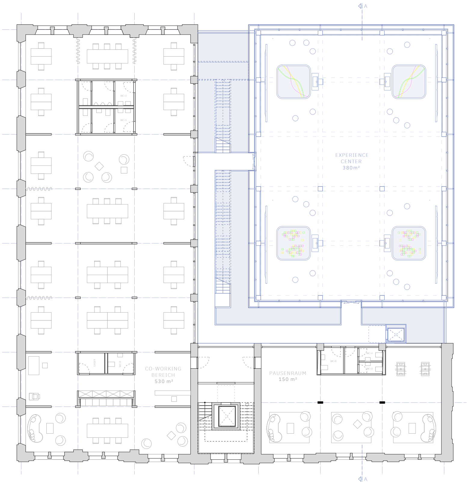
GRUNDRISS - 2. OBERGESCHOSS
