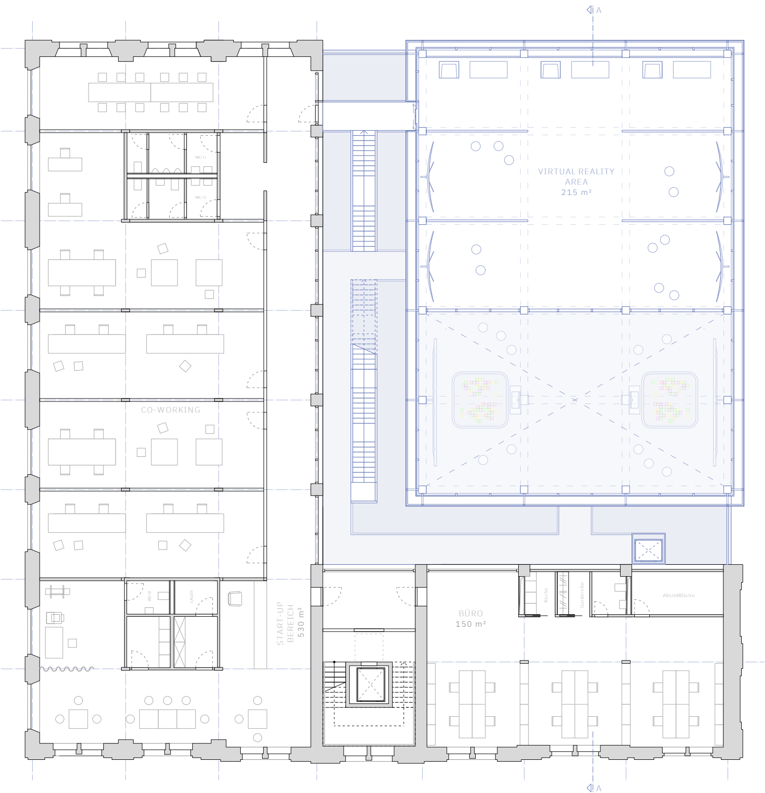
GRUNDRISS - 3. OBERGESCHOSS
