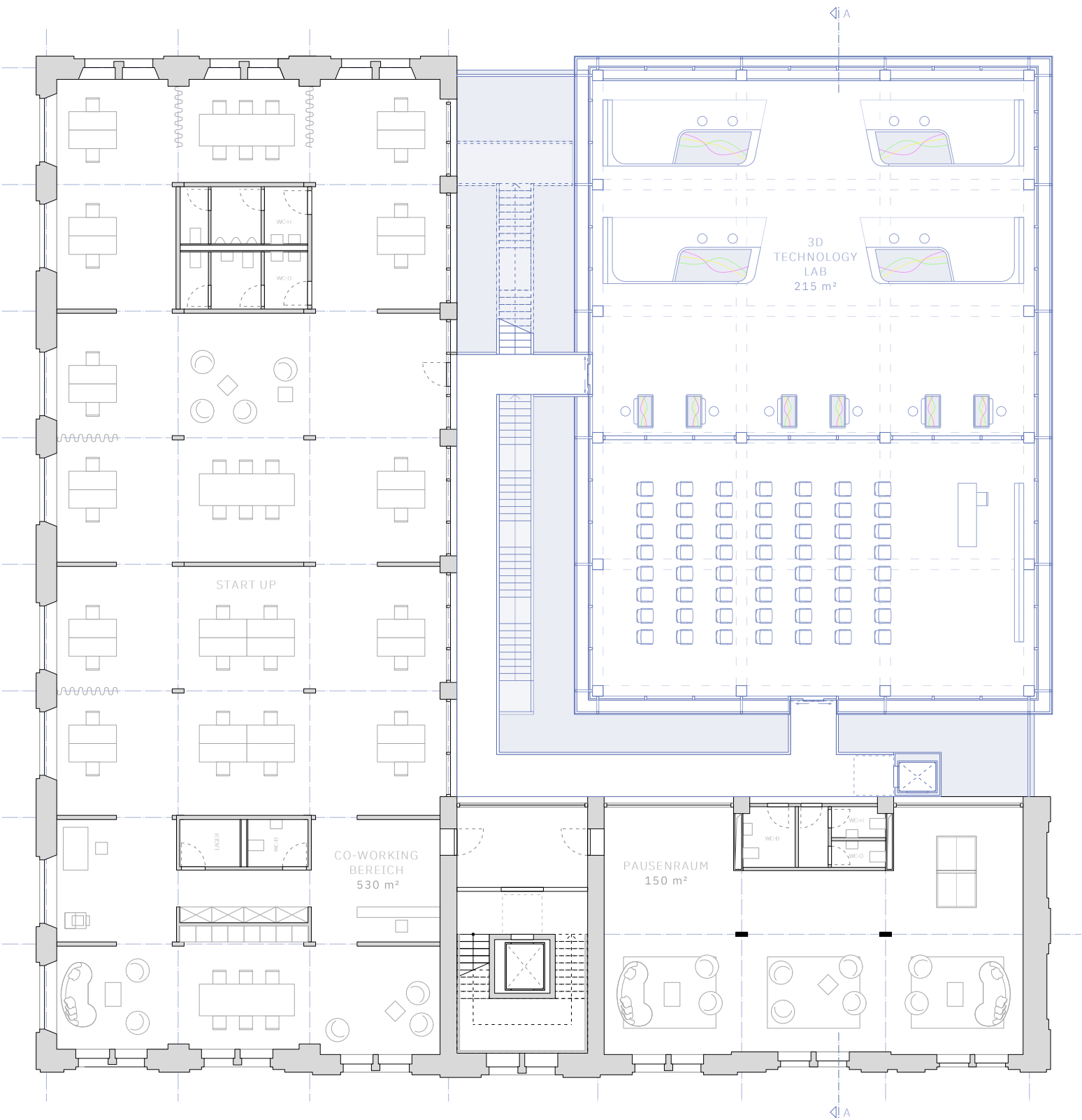
GRUNDRISS - 4. OBERGESCHOSS
