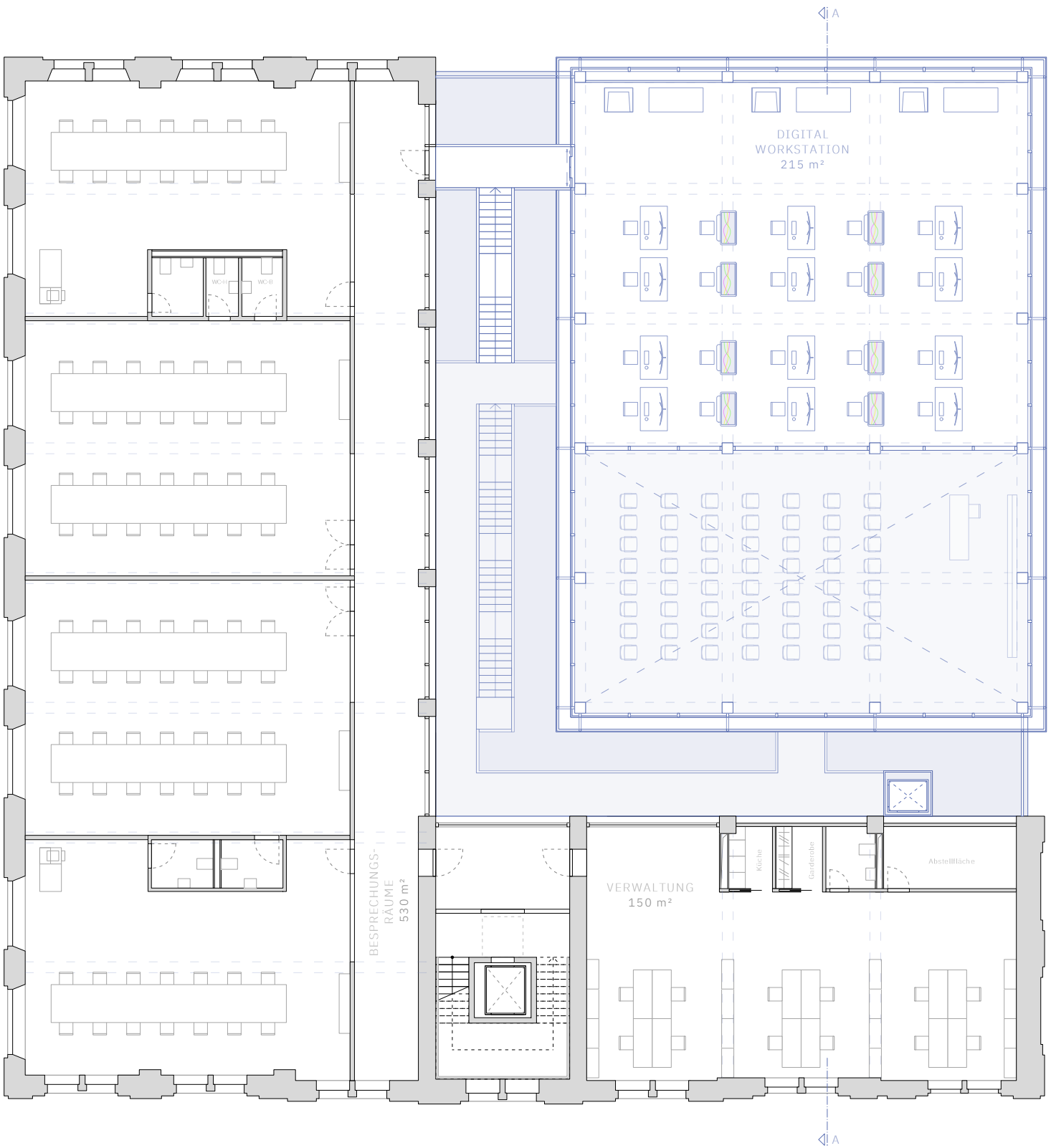
GRUNDRISS - 5. OBERGESCHOSS
