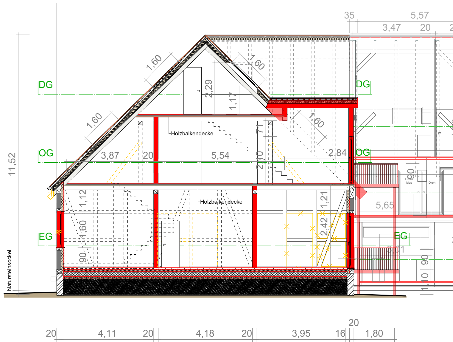
SCHNITT D1 REIHENENDHAUS SCHULWEG 11
