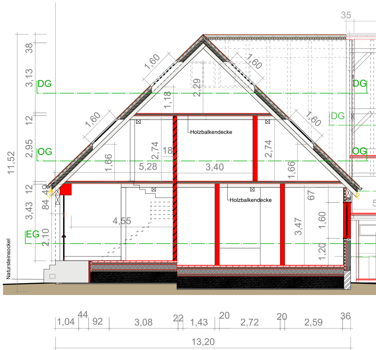
SCHNITT D2 REIHENENDHAUS SCHULWEG 11
