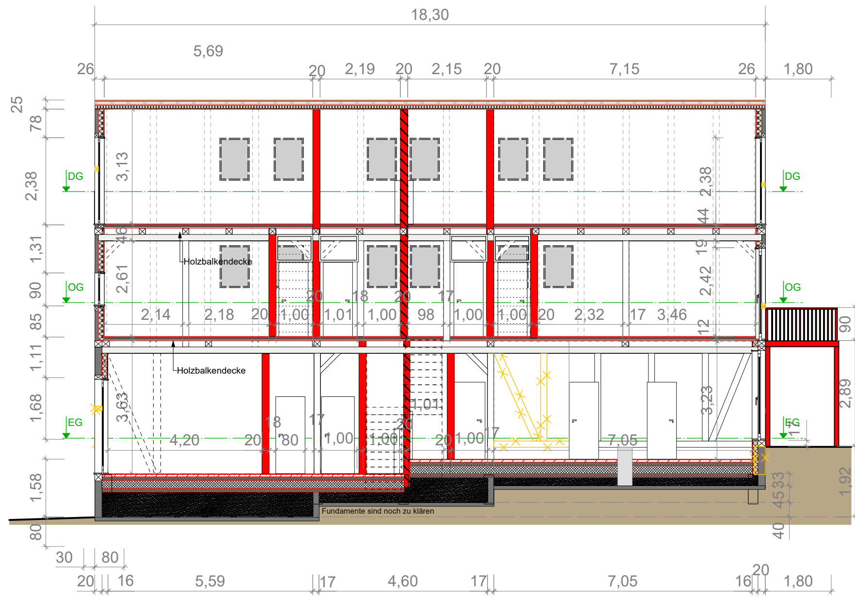
SCHNITT C REIHENENDHAUS SCHULWEG 11
