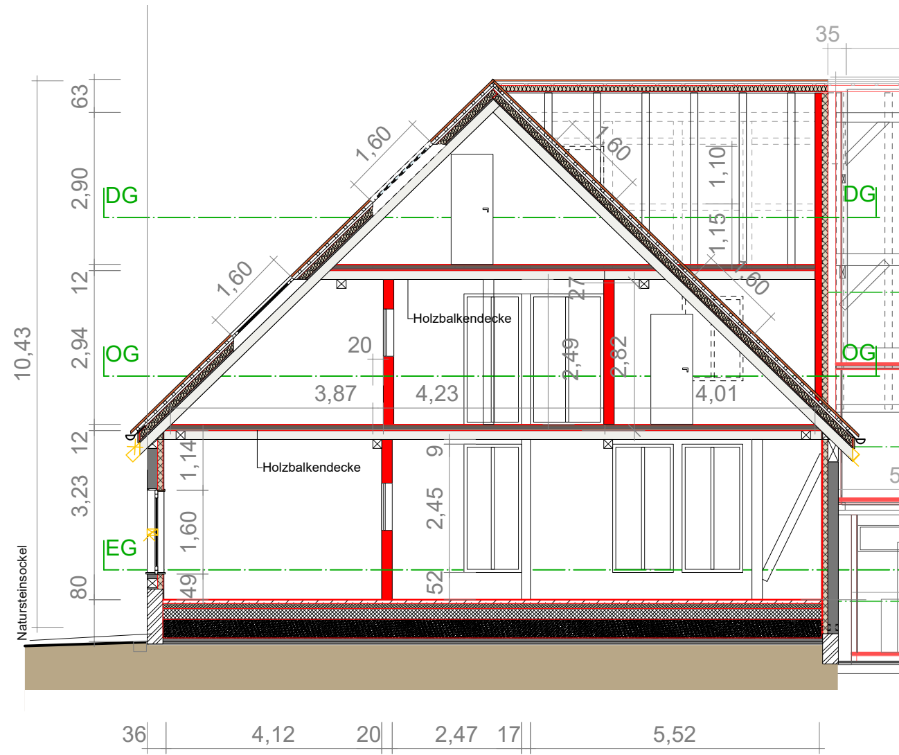
SCHNITT D3 REIHENENDHAUS SCHULWEG 11
