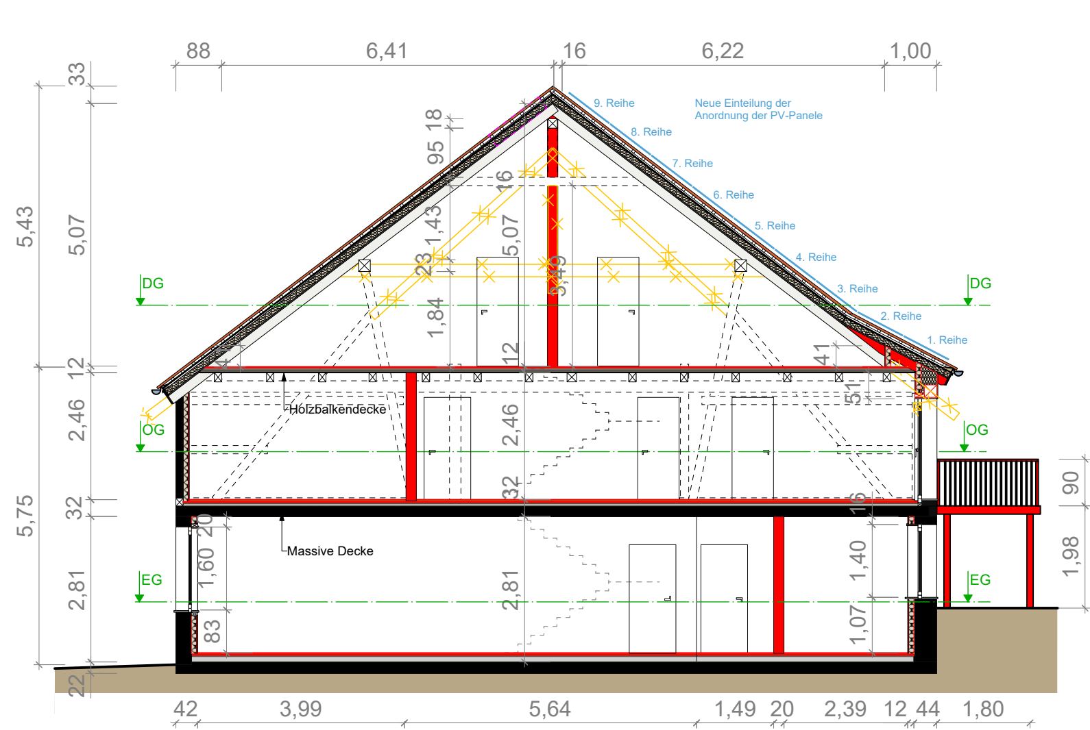
SCHNITT A.3 REIHENMITTELHAUS 6B
