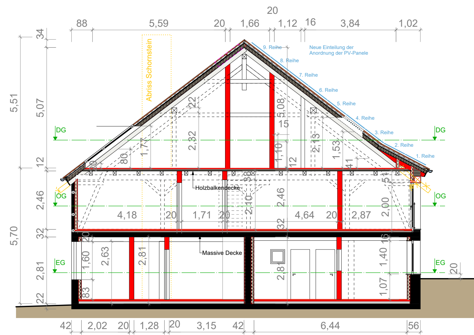
SCHNITT A.2 REIHENENDHAUS 6A
