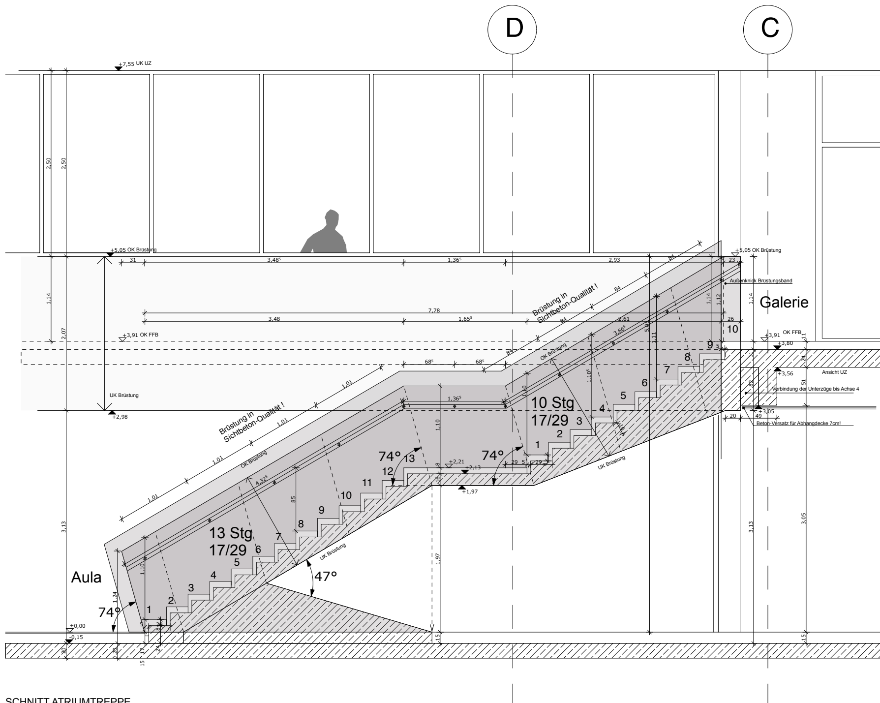
SNITT ATRIUMTREPPE
