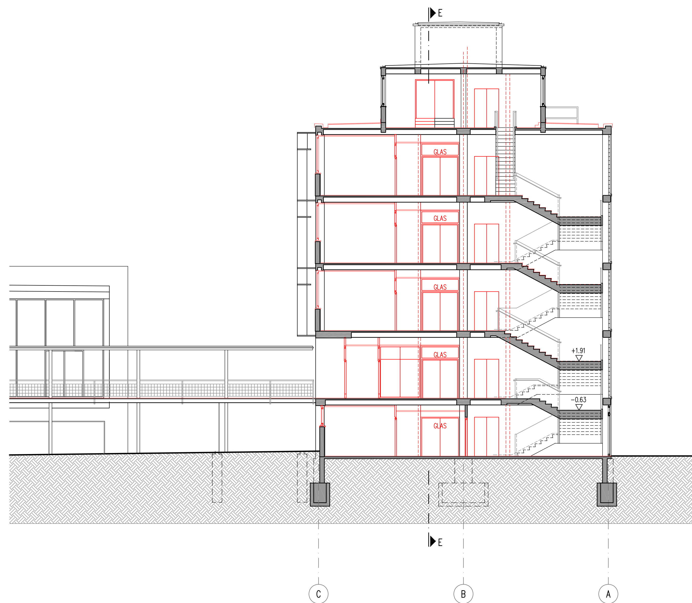
SCHNITT C-C
