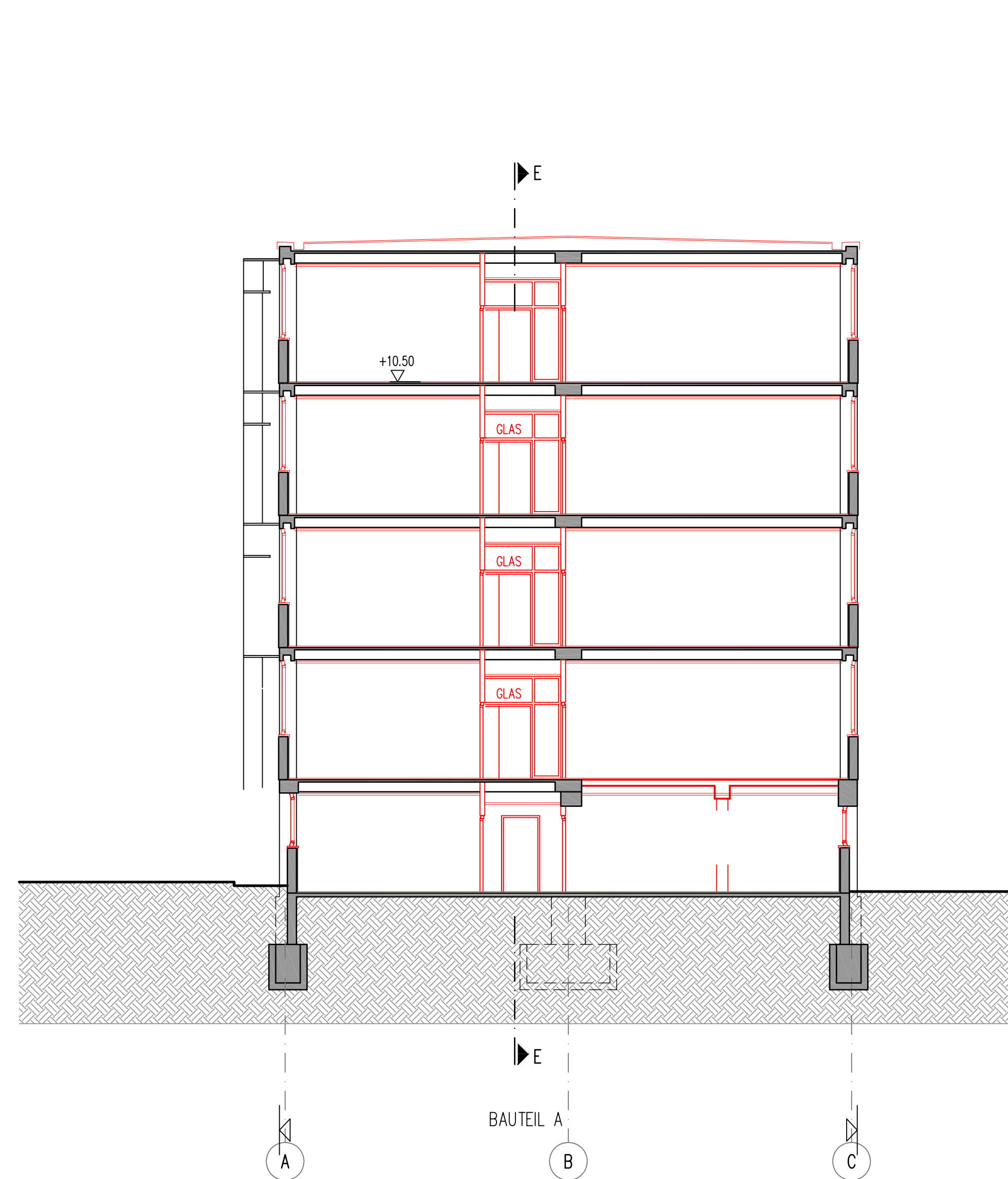
SCHNITT F-F
