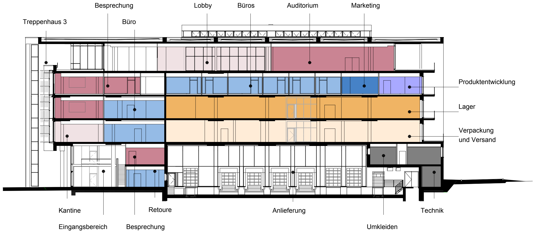
Querchnitt Anlieferungsbereich
