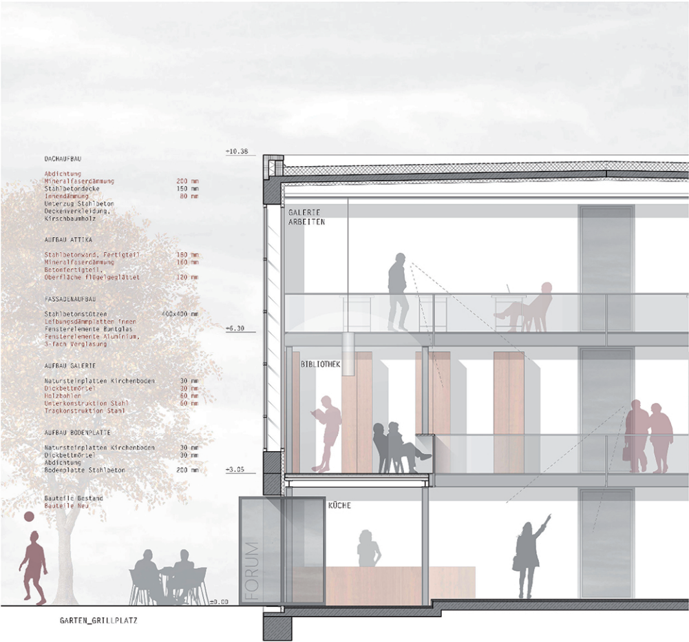
FASSADENSCHNITT BESTAND _ M 1:50
