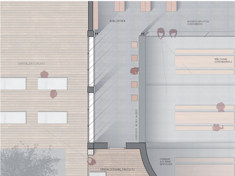
TEILGRUNDRISS BESTAND _ M 1:50
