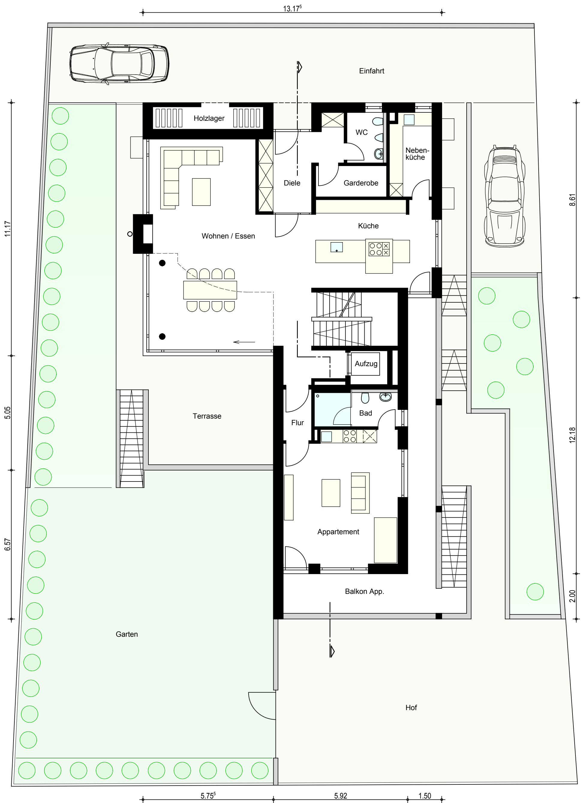
Erdgeschoss
