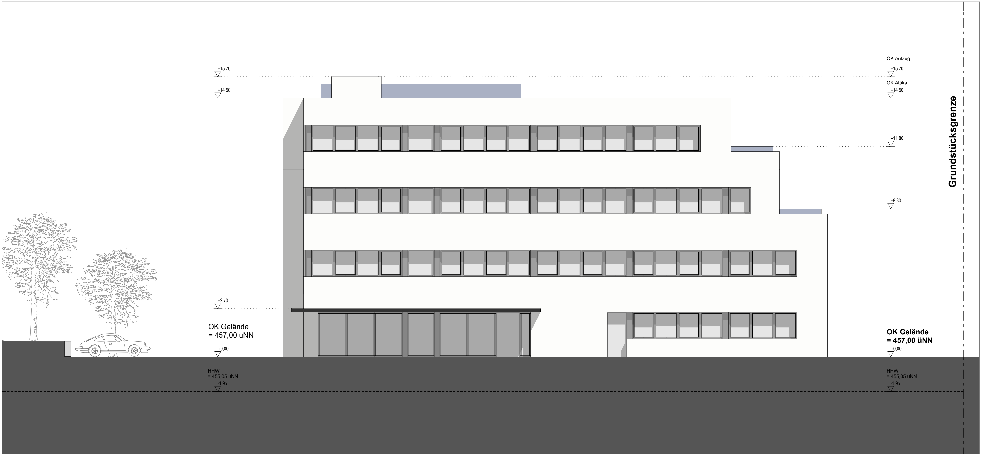
Ansicht Nord M 1/100
