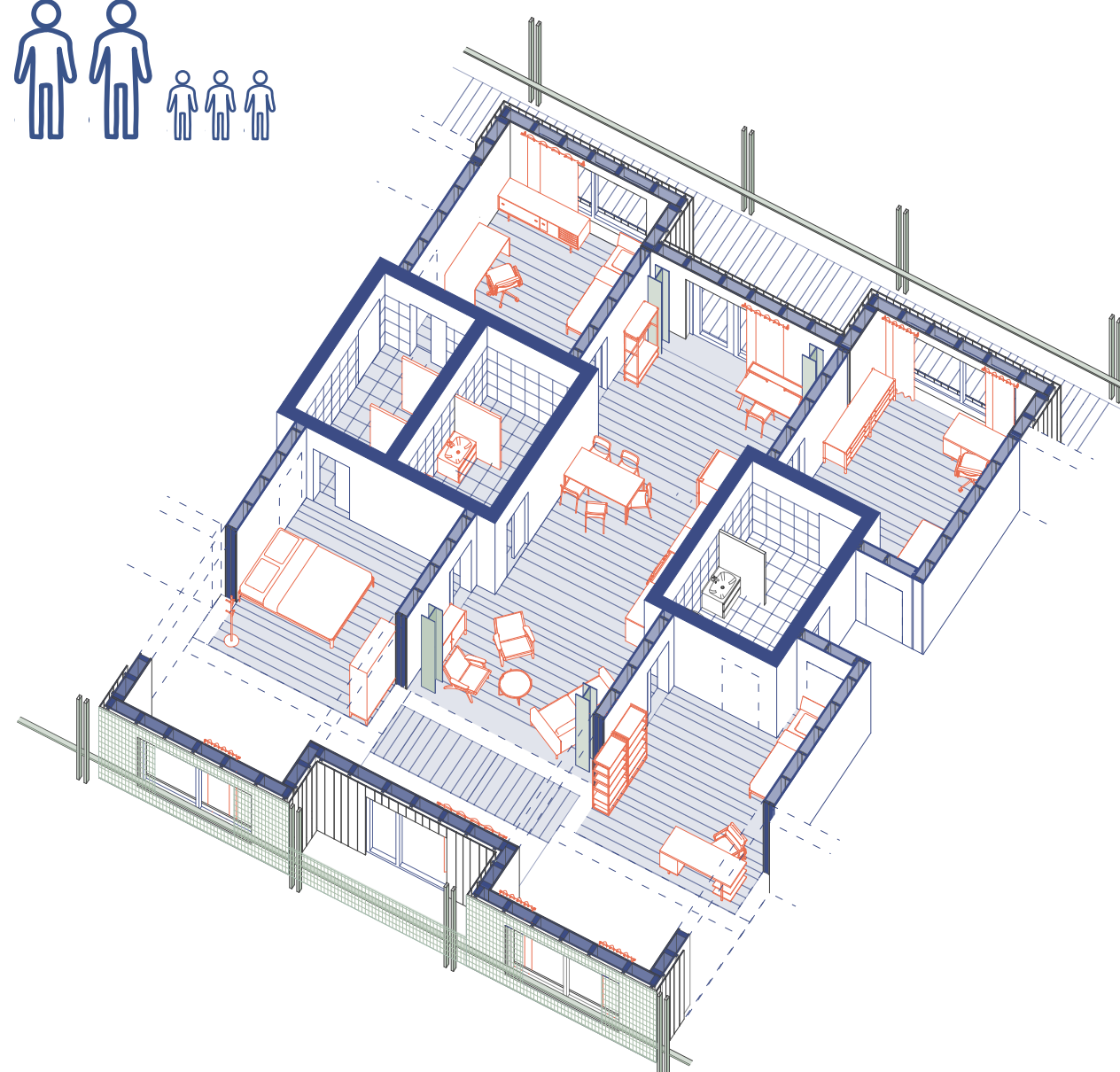
Größtmögliche Wohneinheit Eine Wohnung (105m²) für 4 -5 Personen. Mit den Schaltzimmern wurde auch ein Badezimmer hinzugefügt.
