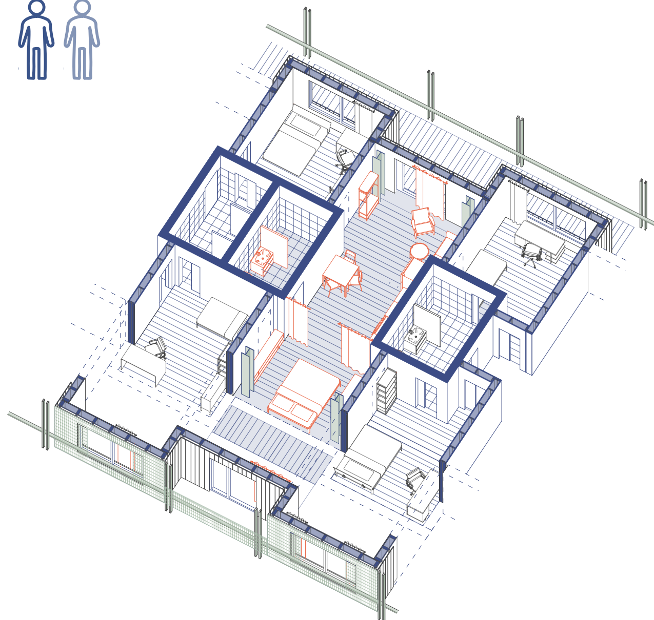
Kleinstmögliche Wohneinheit Eine Wohnung (42m²) für 1-2 Personen. Falls sich die Bedürfnisse ändern können in Zukunft bis zu 4 Schlafzimmer und ein Bad hinzugefügt werden.
