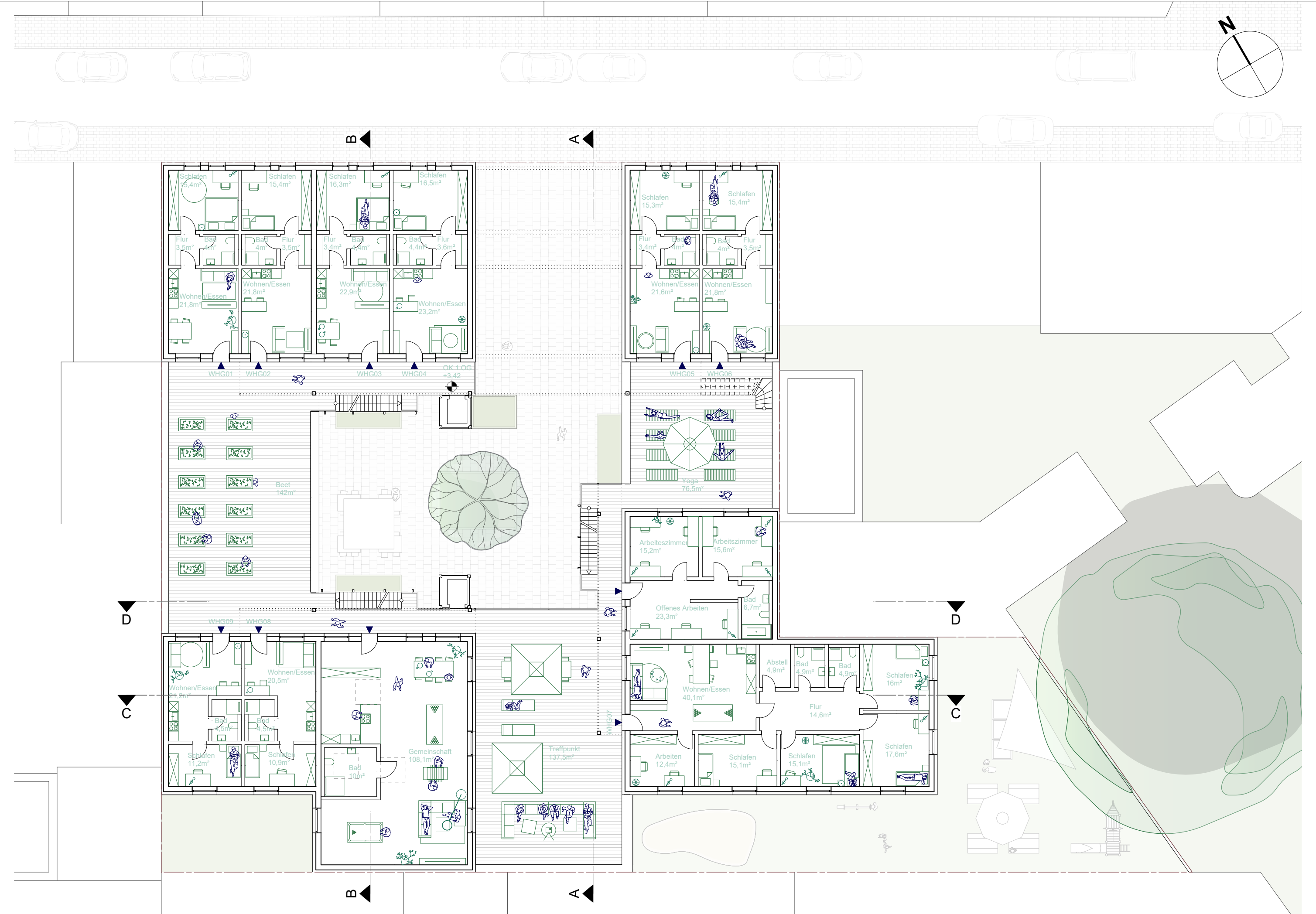
GRUNDRISS 1.OG
