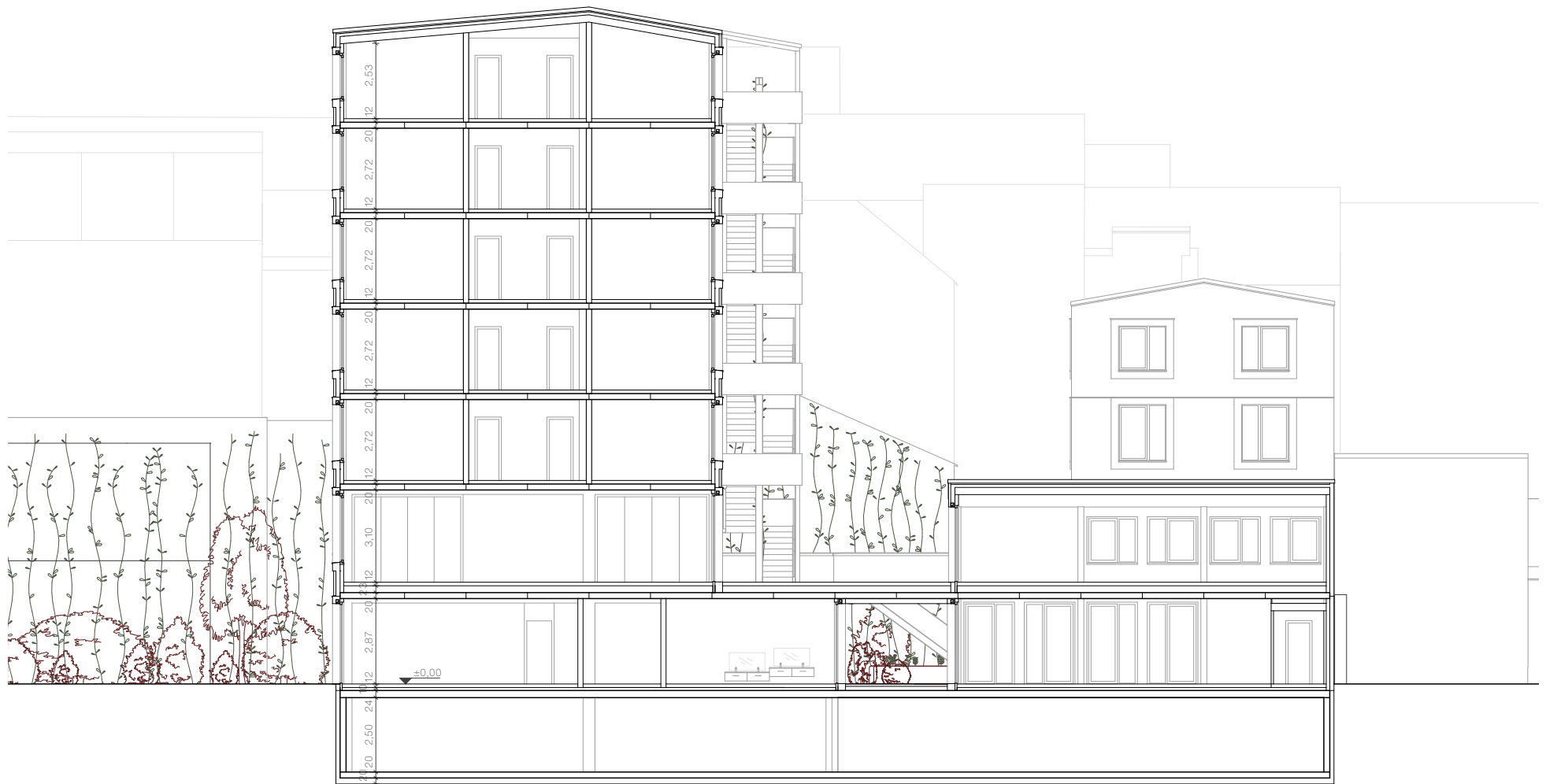
Schnitt AA 1:200
