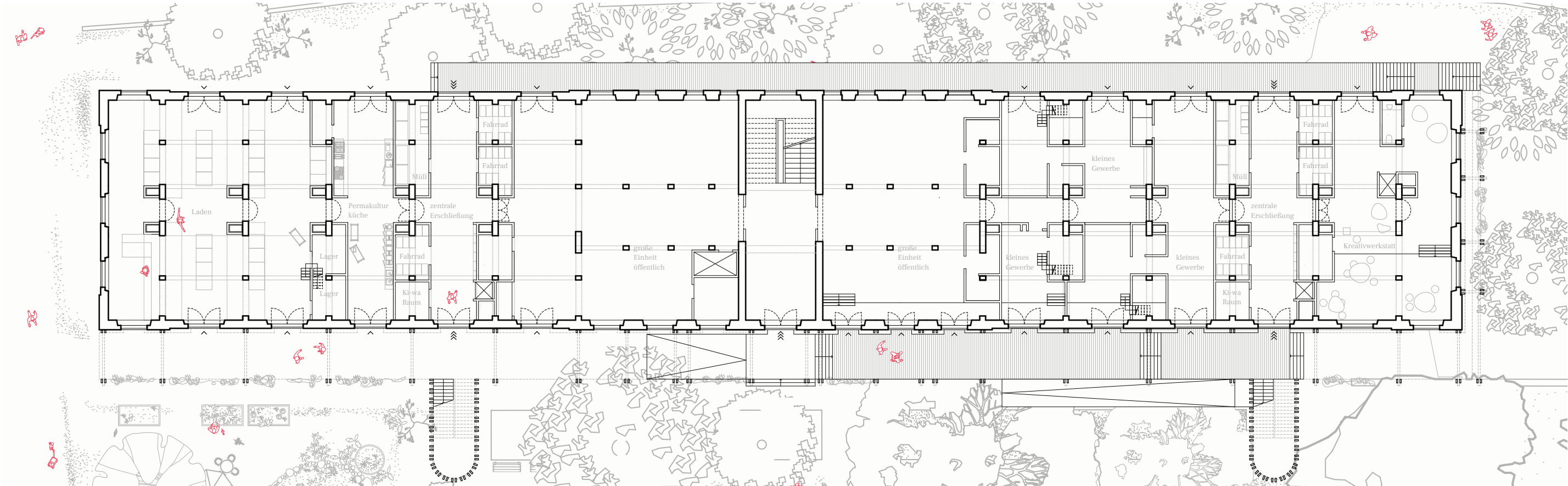
ERDGESCHOSS
