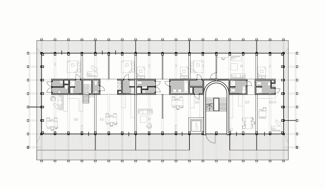
REGELGESCHOSS
