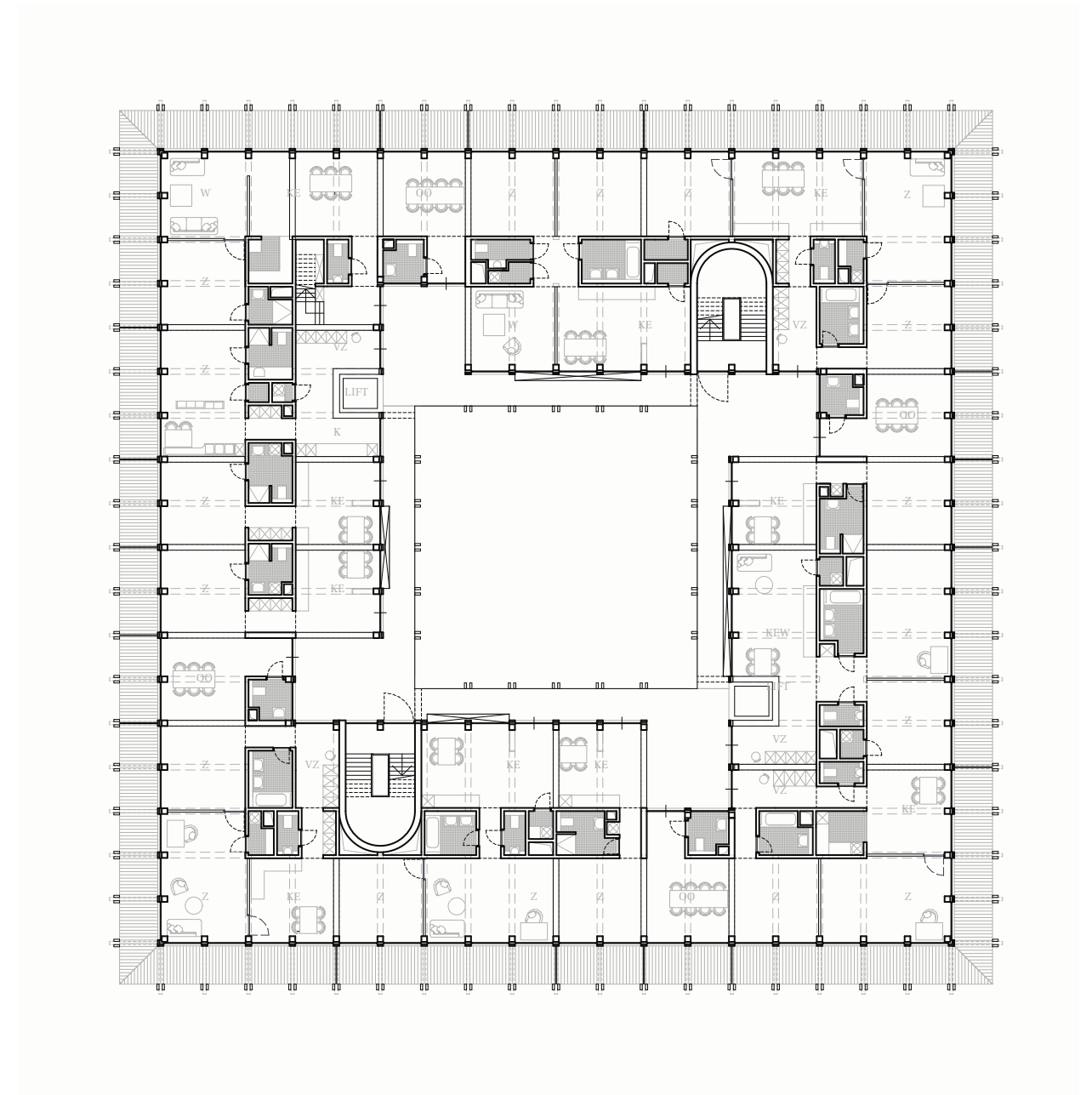
REGELGESCHOSS
