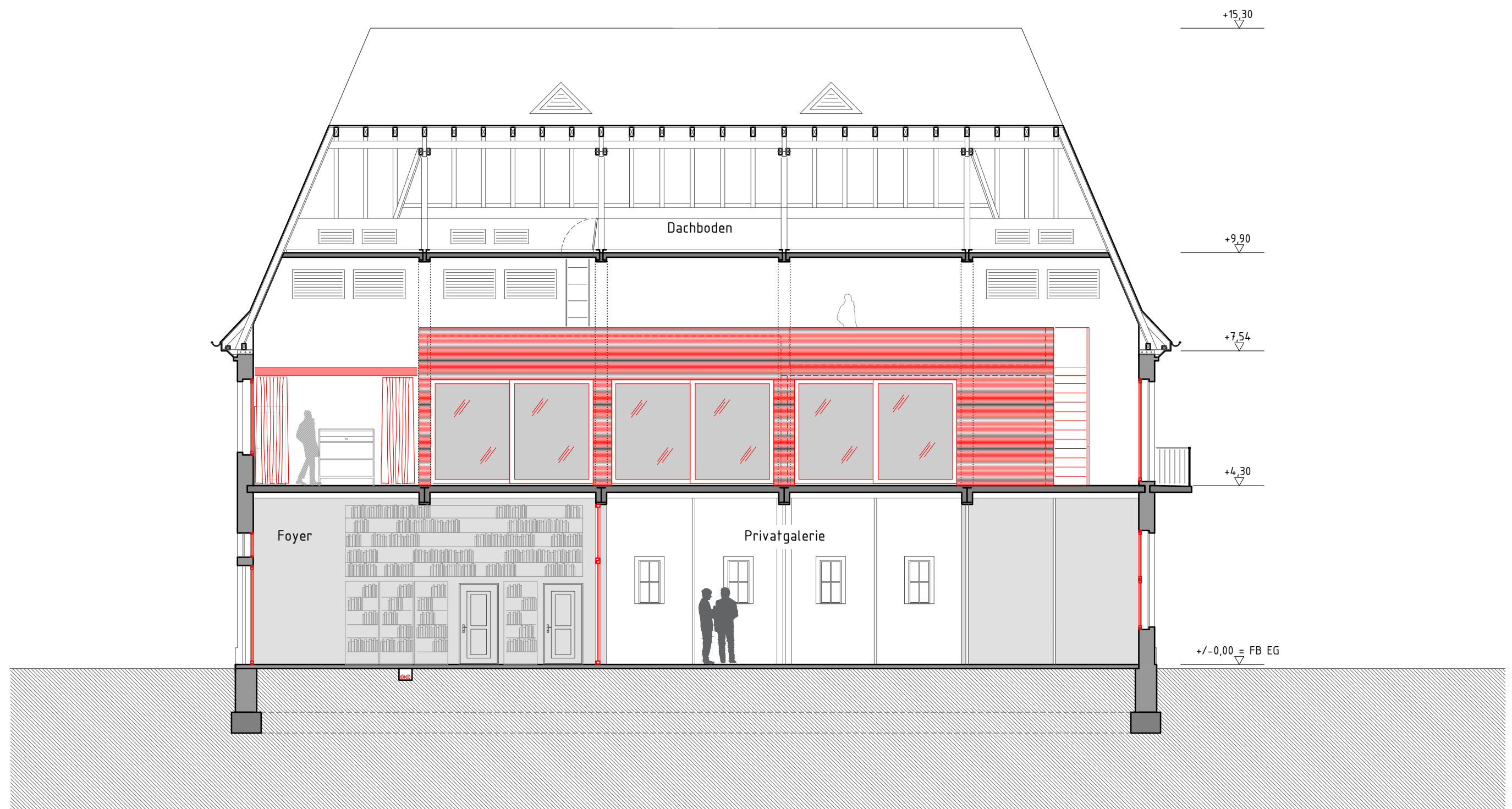
Schnitt CC M 1:100
