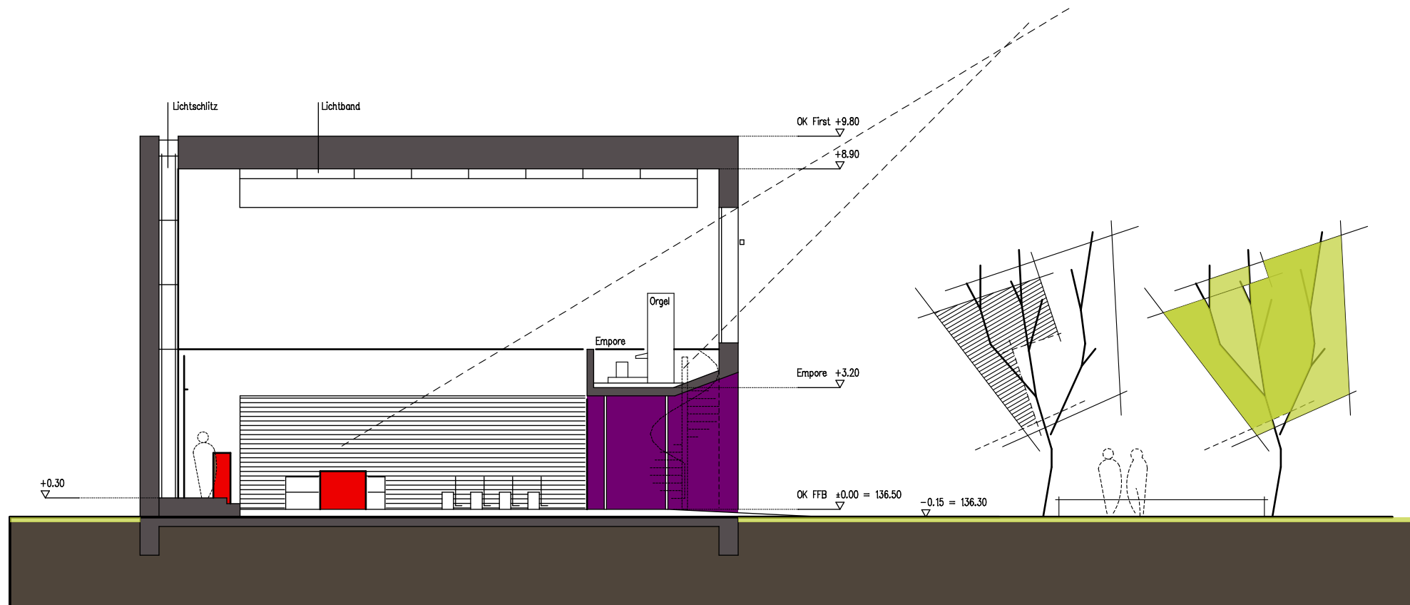
SCHNITT B-B
