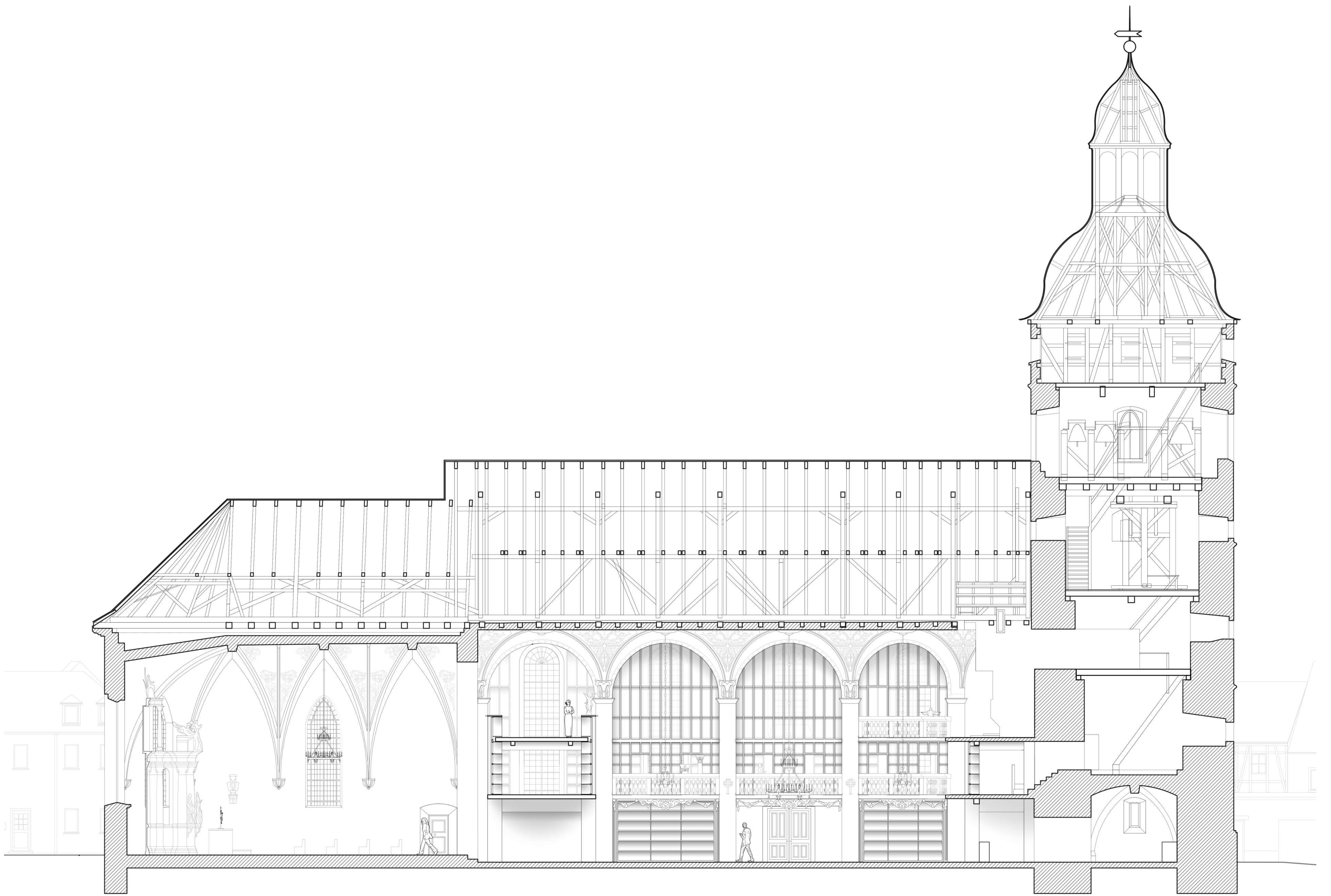
Längsschnitt M1:100
