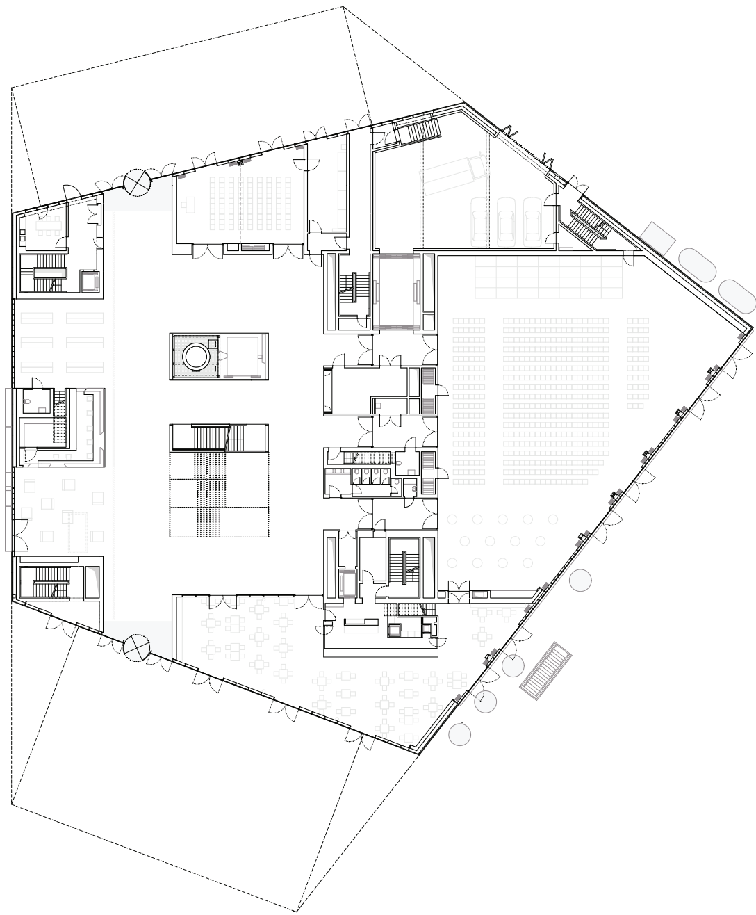
Erdgeschoss 1:500
