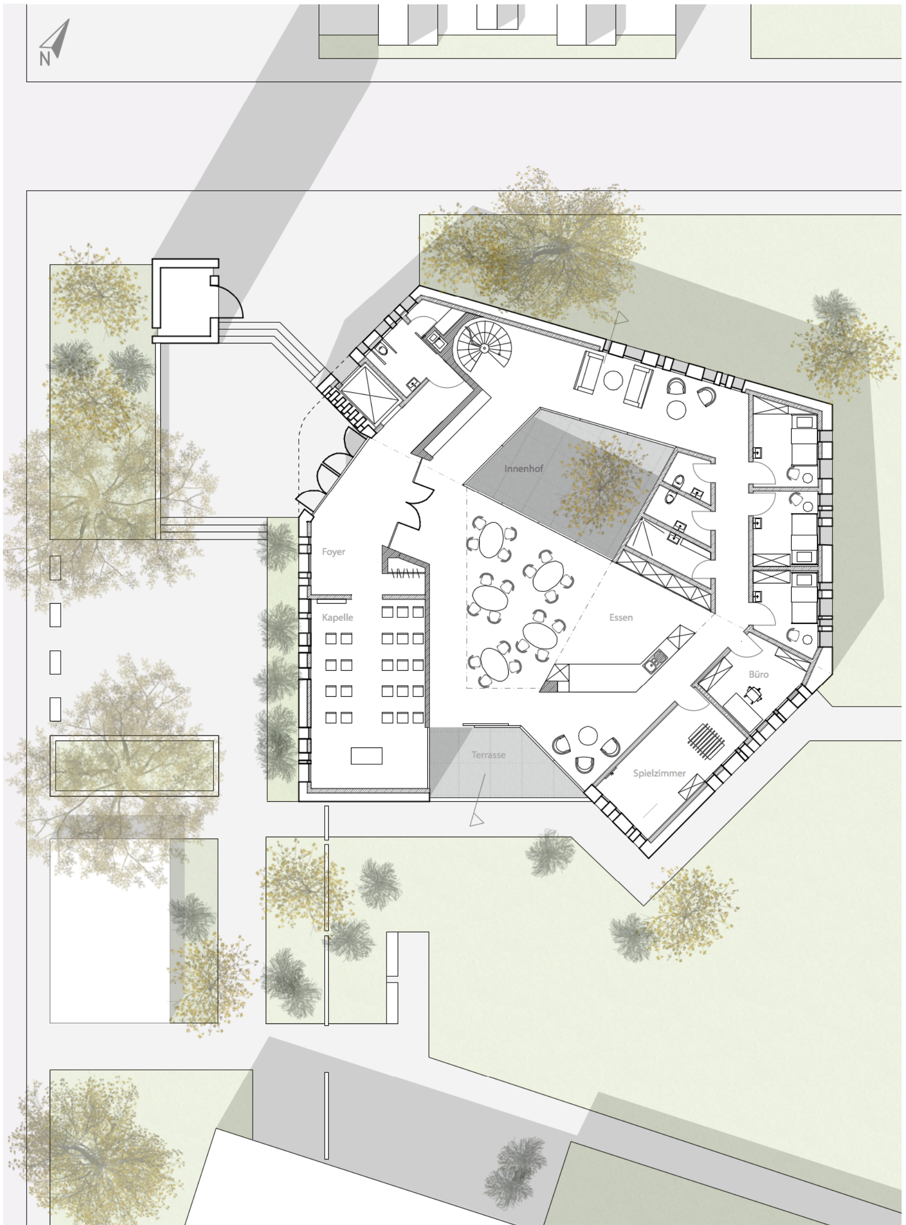
Erdgeschoss
