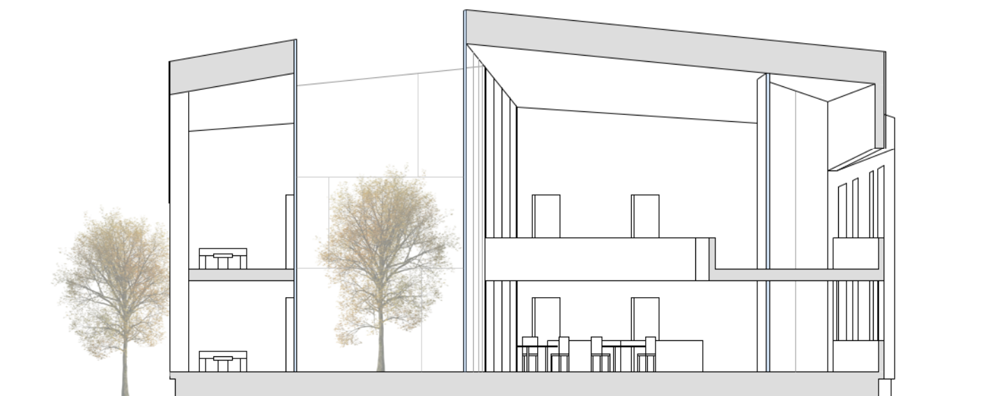
Schnitt
