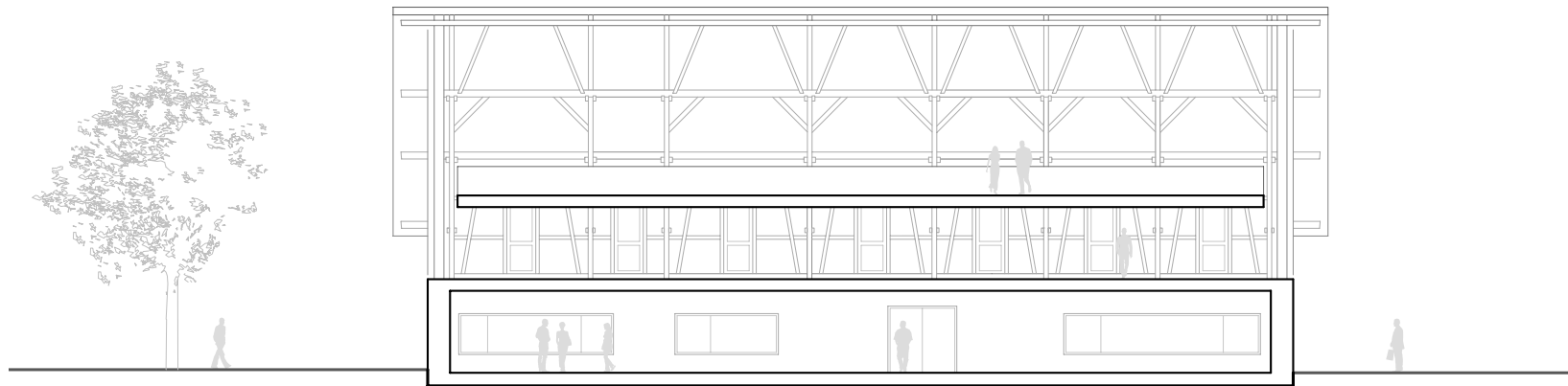
längsschnitt
