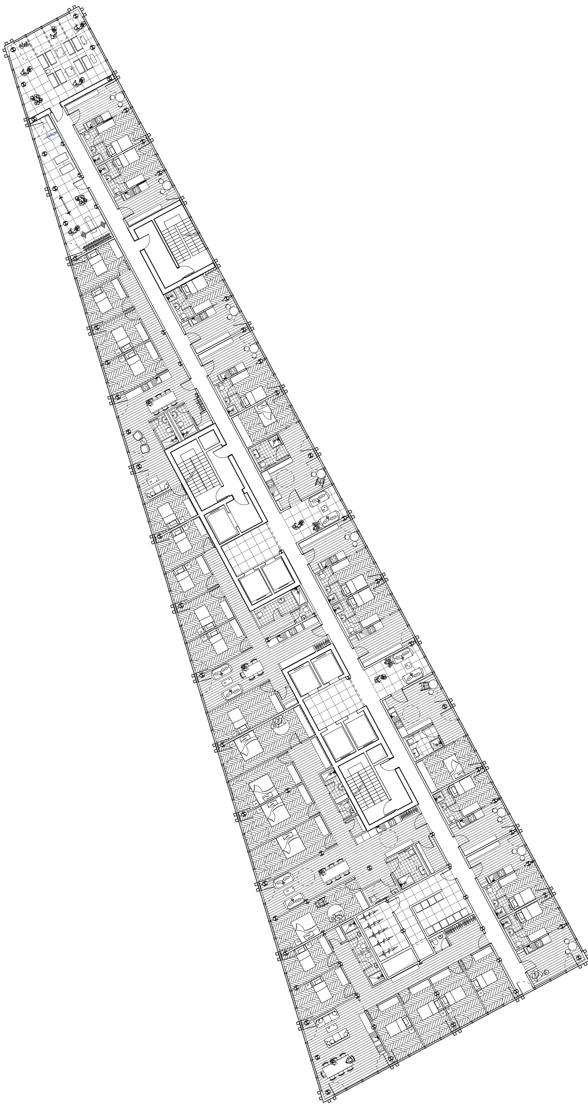
Grundriss 16. - 30. OG 1/200
