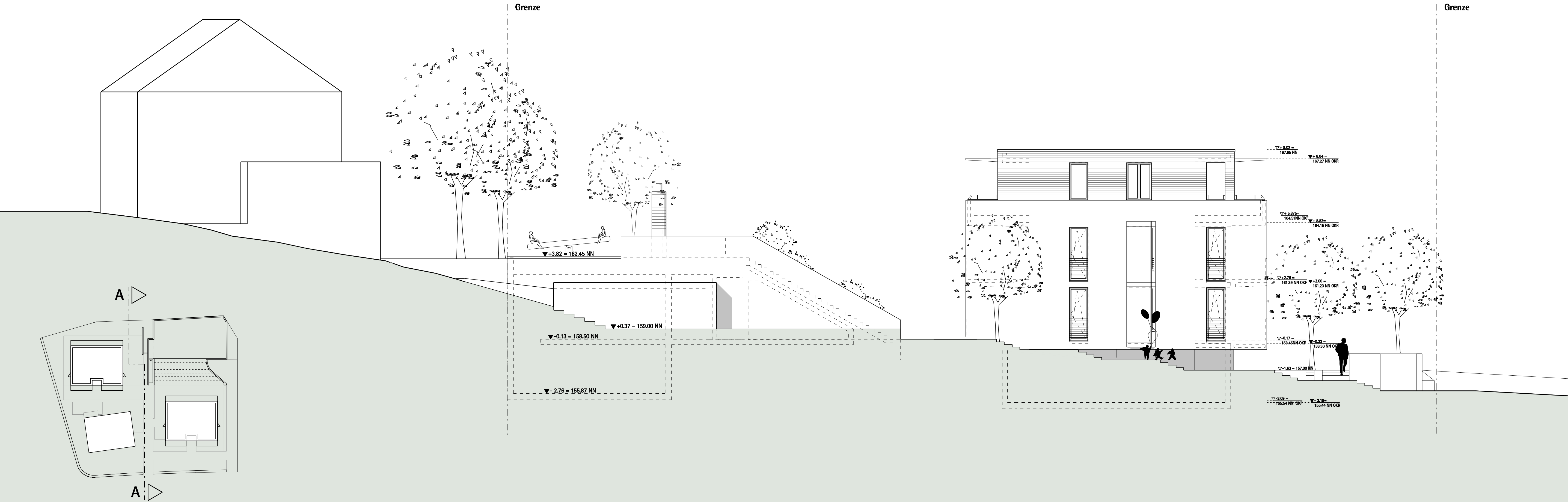
Schnitt A-A
