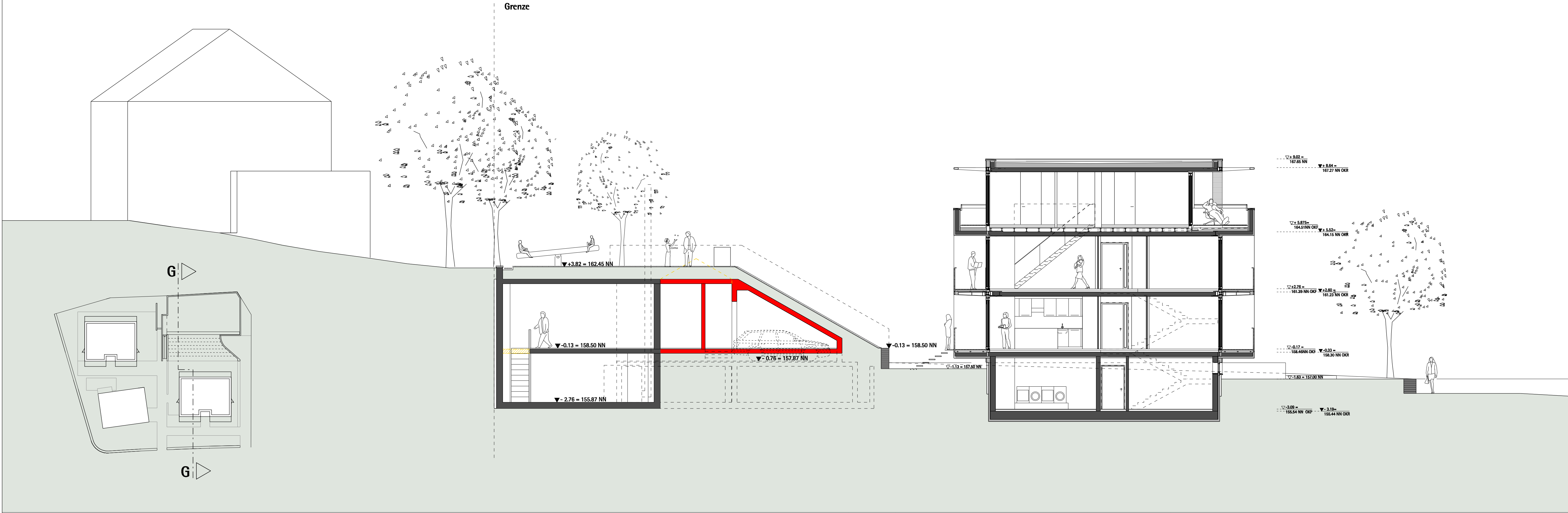
Schnitt G-G
