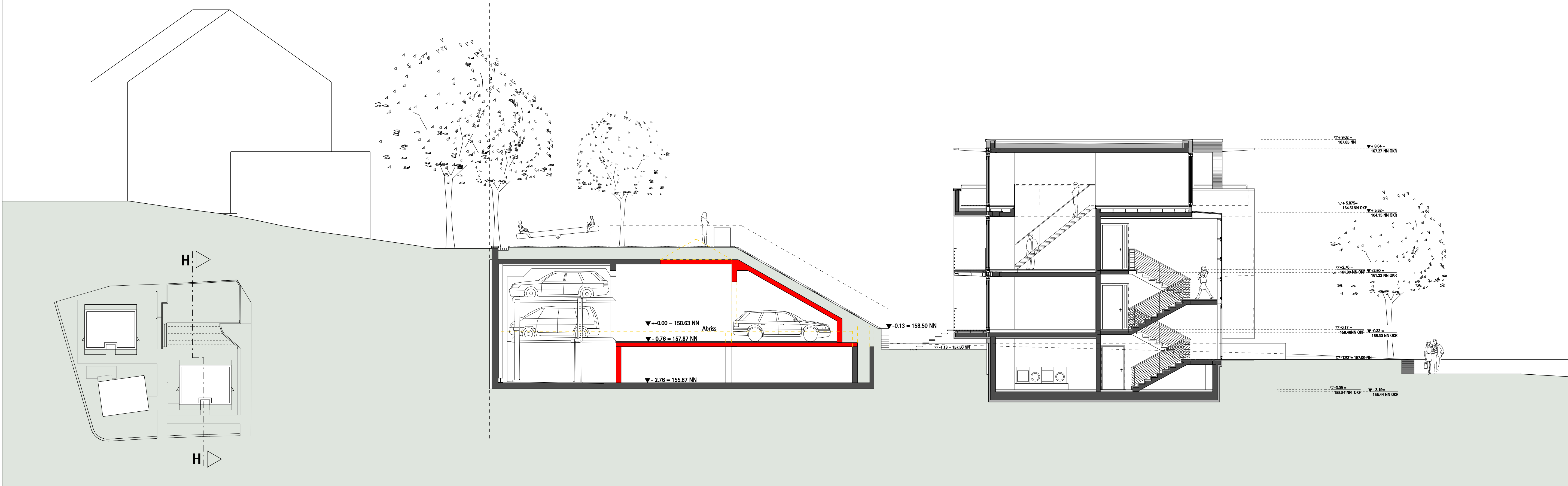
Schnitt H-H
