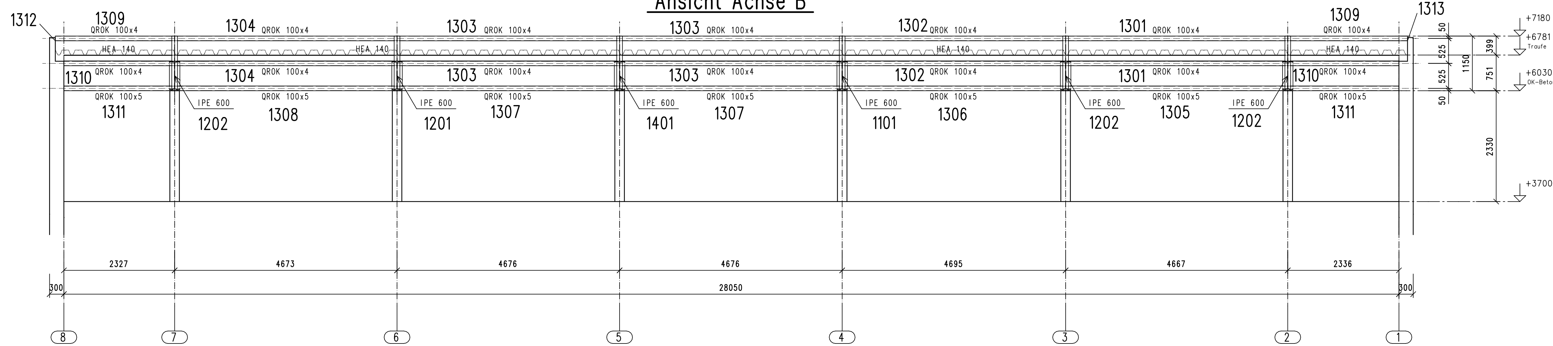
Ansicht Achse B
