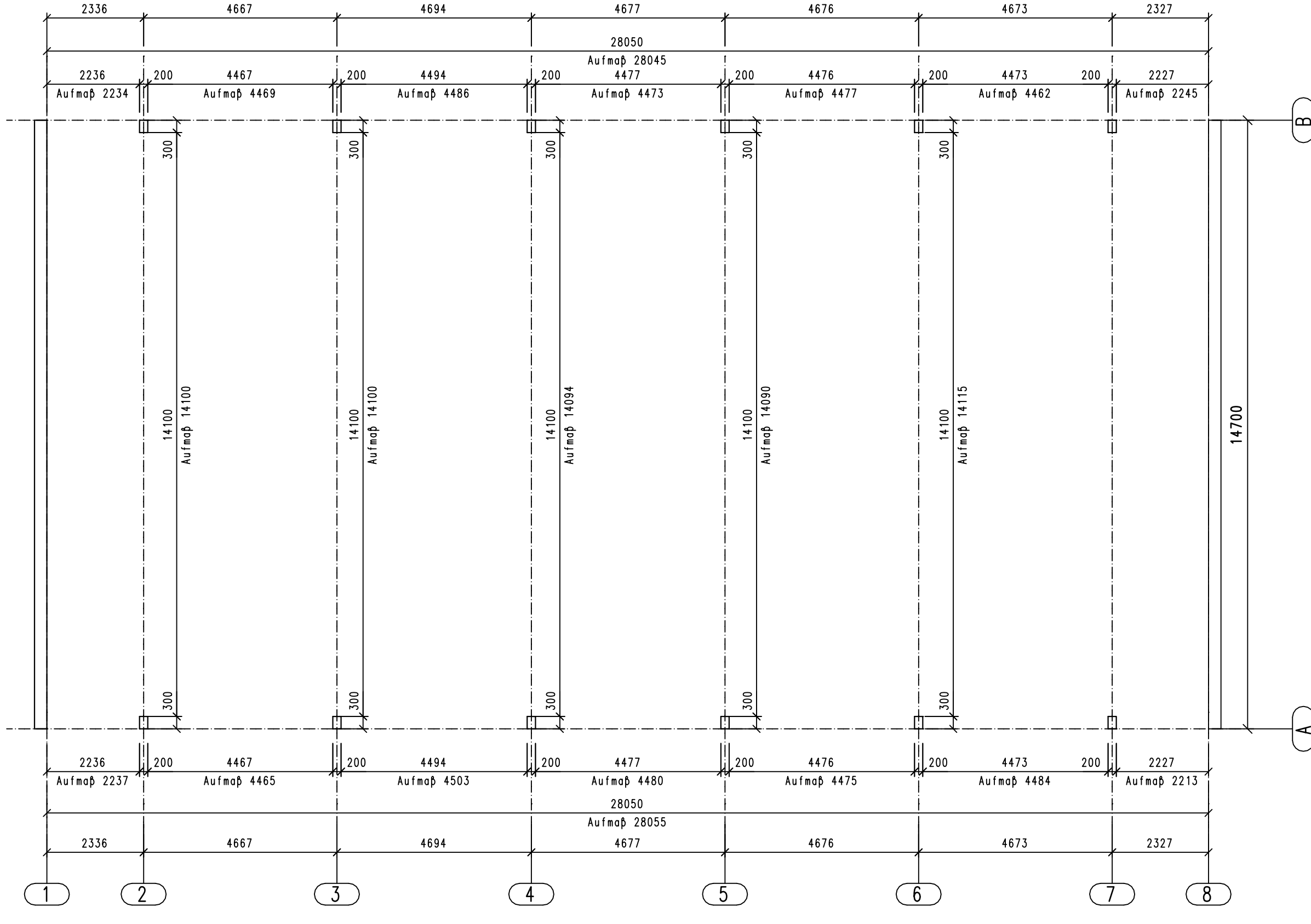
Aufmaß und Festlegung der Achsmaße und Einteilung M 1:100
