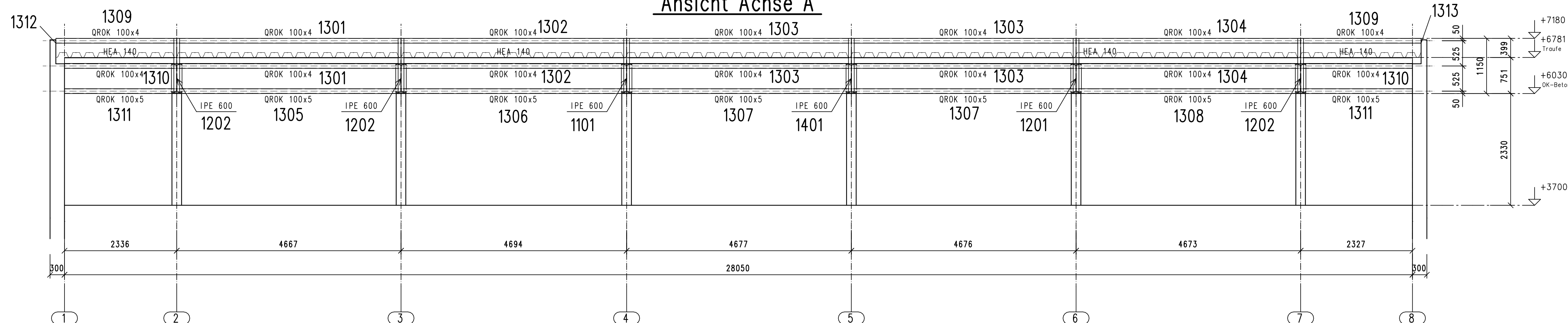
Ansicht Achse A
