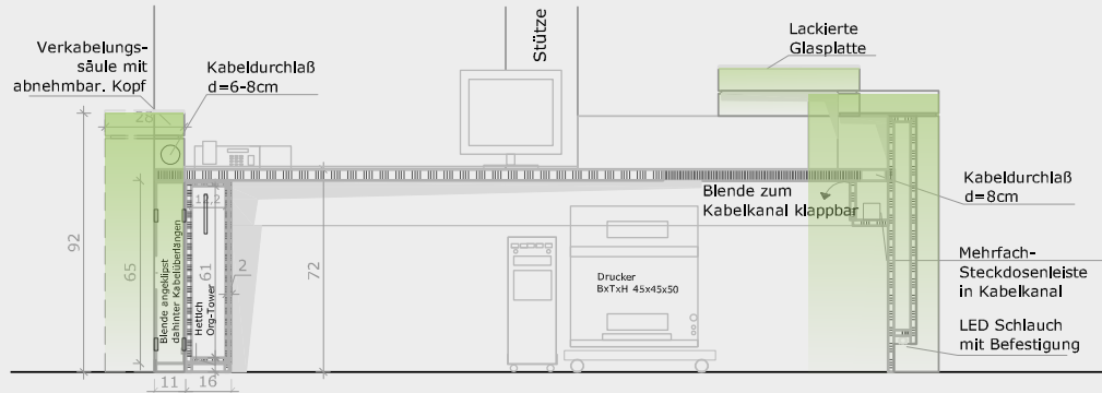
Vertikalschnitt A-A Empfangstheke
