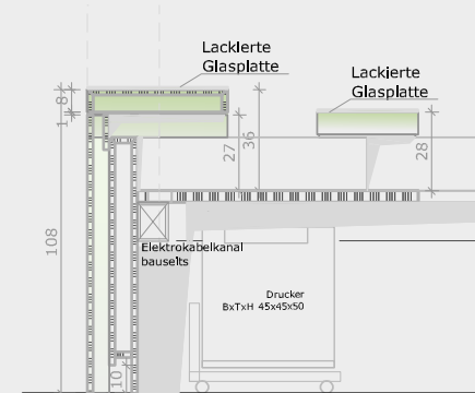
Vertikalschnitt B-B Empfangstheke
