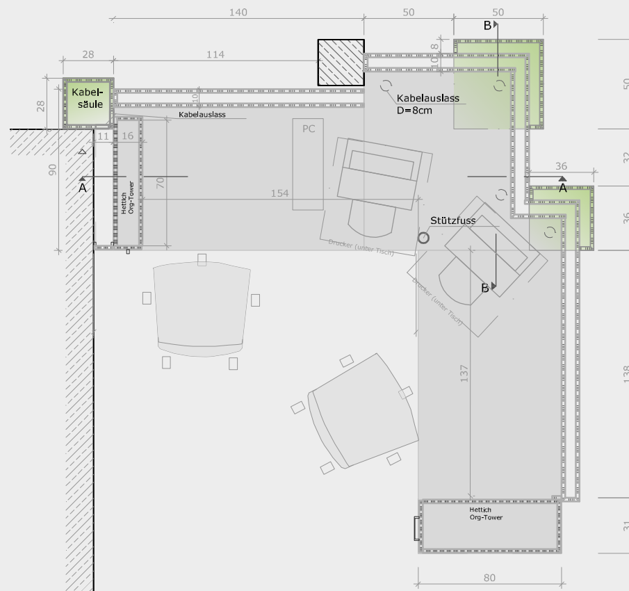
Draufsicht / Horizontalschnitte Empfangstheke
