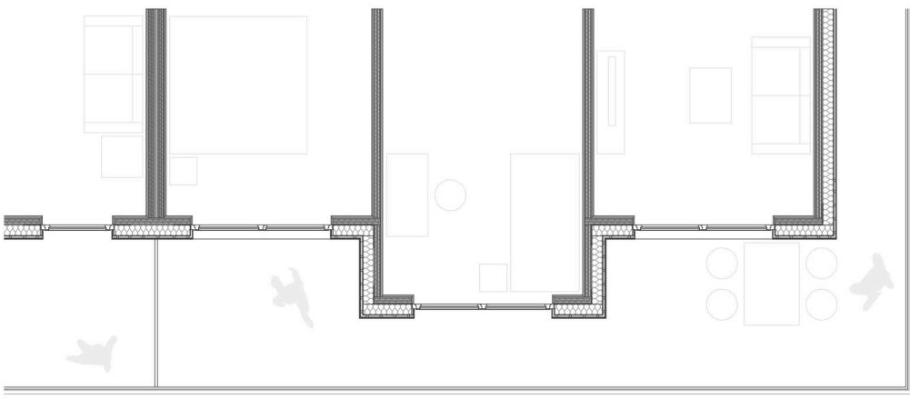
Teilgrundriss M 1:50
