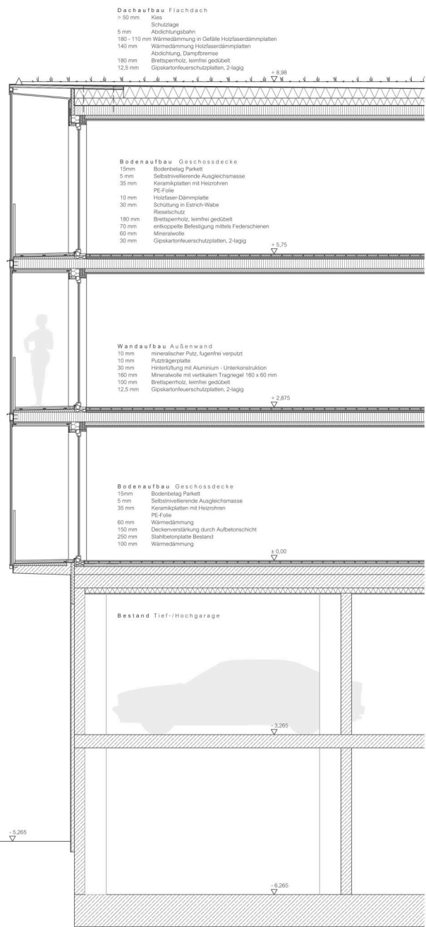
Teilschnitt M 1:50
