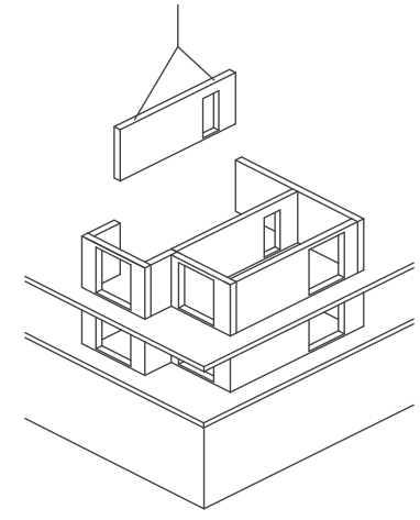
Axonometrie Konstruktion
