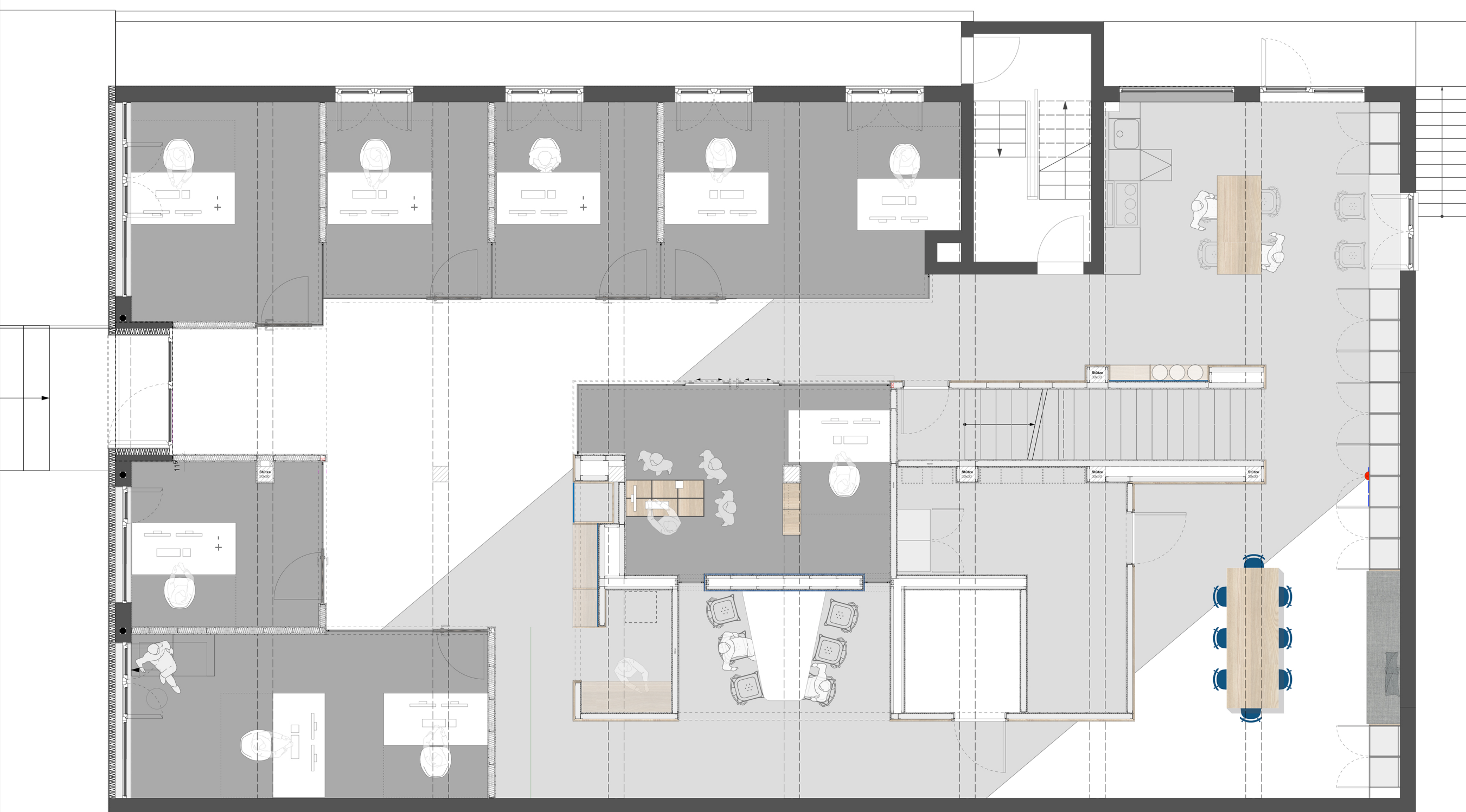
GRUNDRISS ERDGESCHOSS
