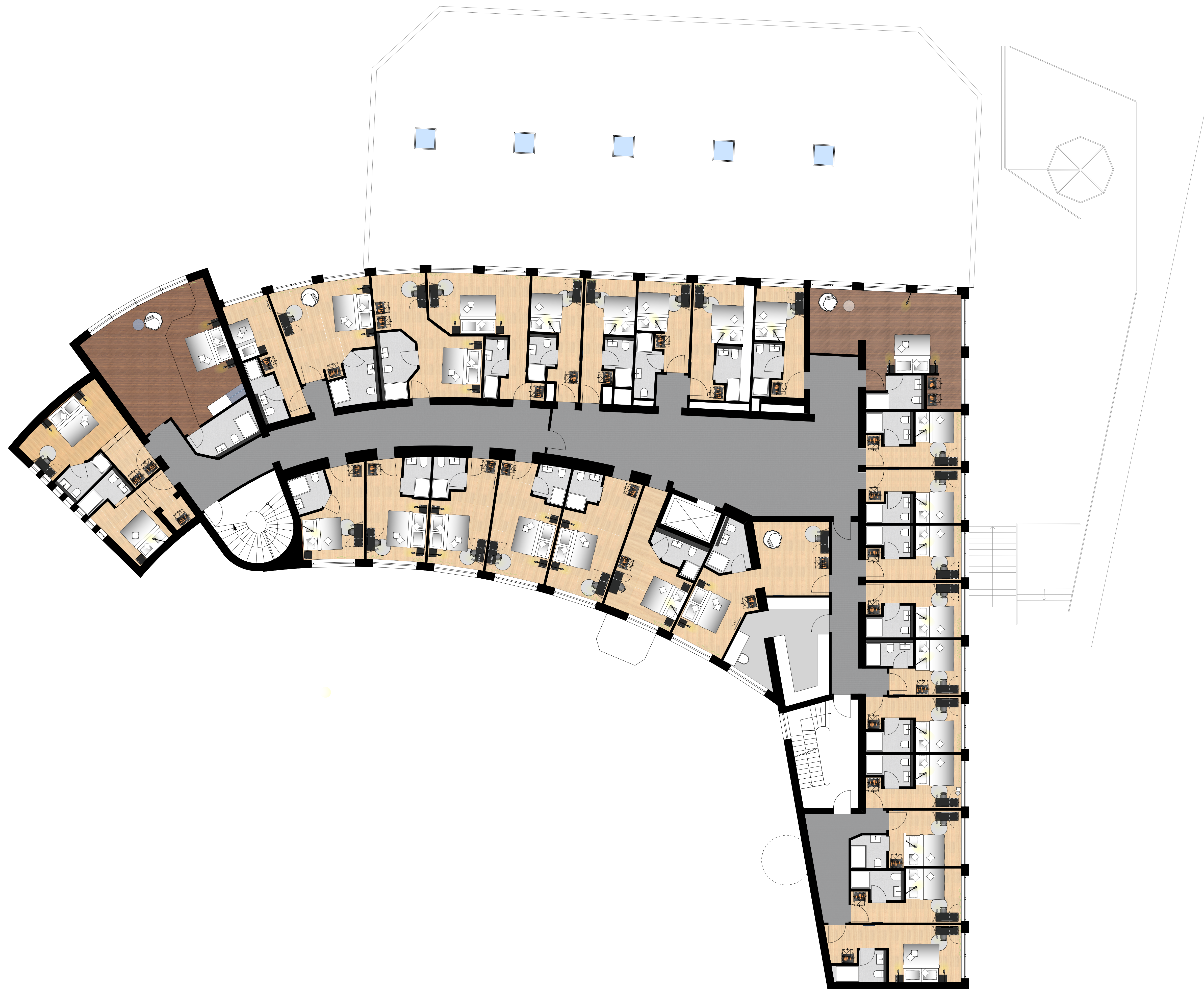
Grundriss 1. Obergeschoss
