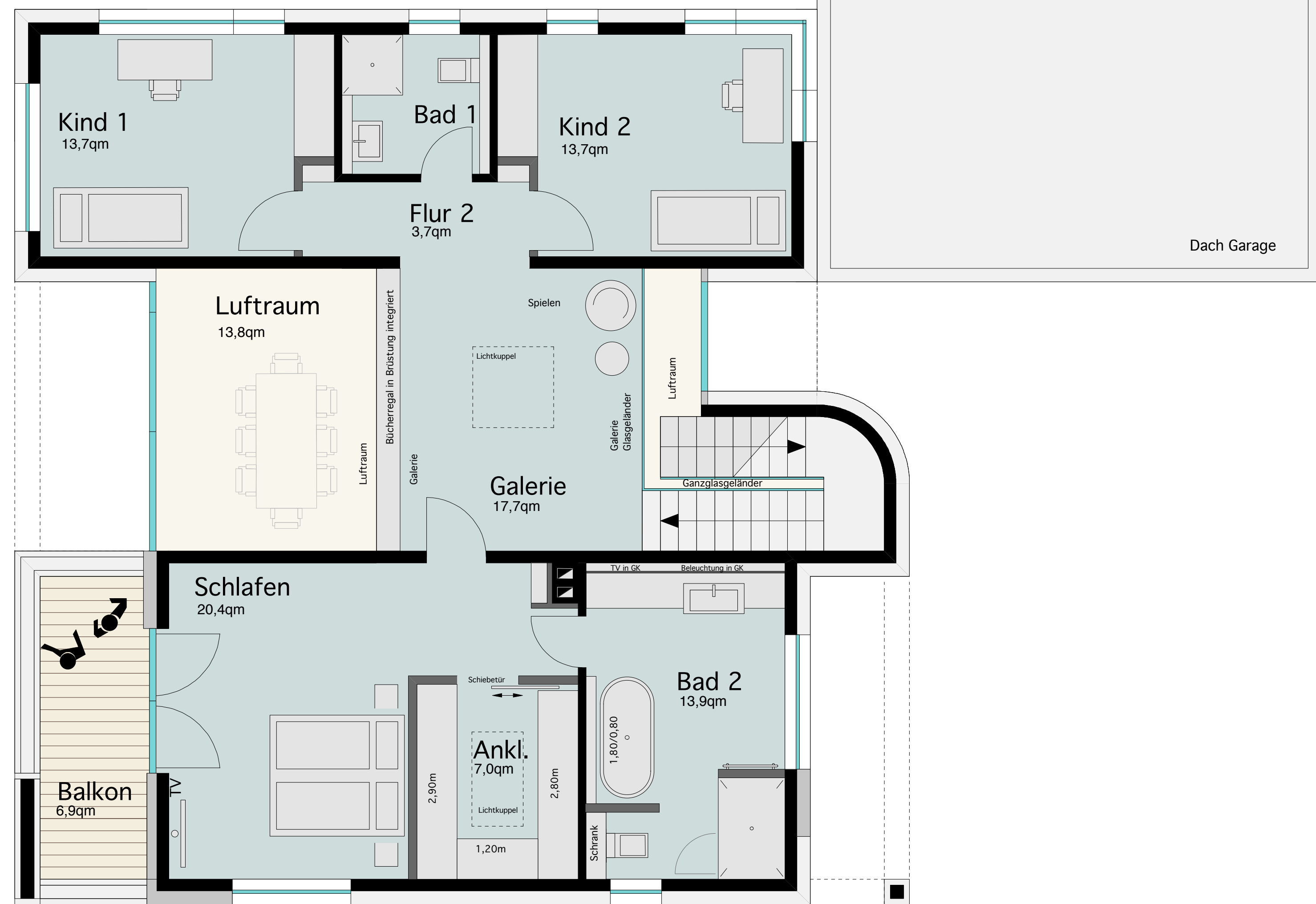
grundriss 1.og
