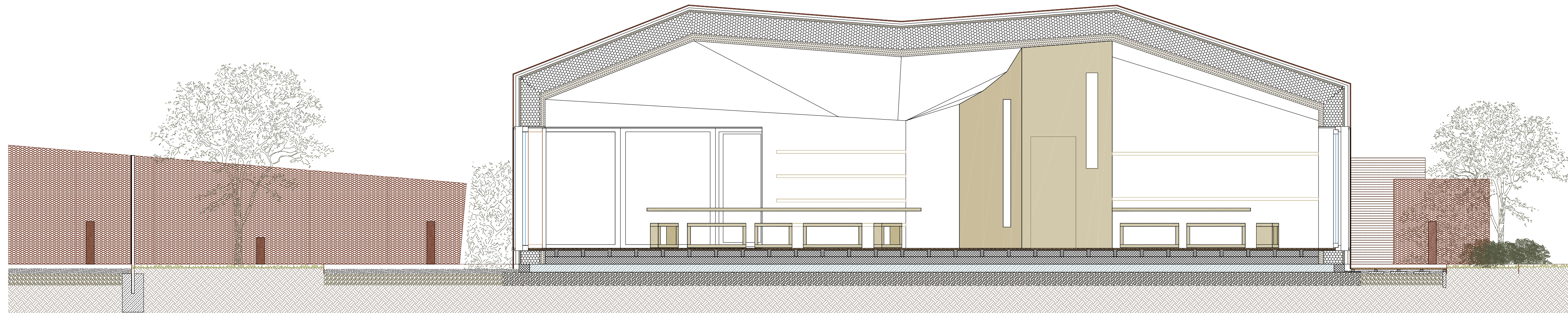
schnitt A-A m 1:50
