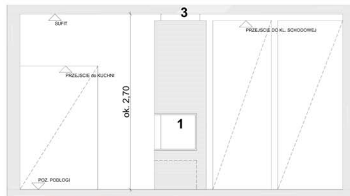
widok frontalny
