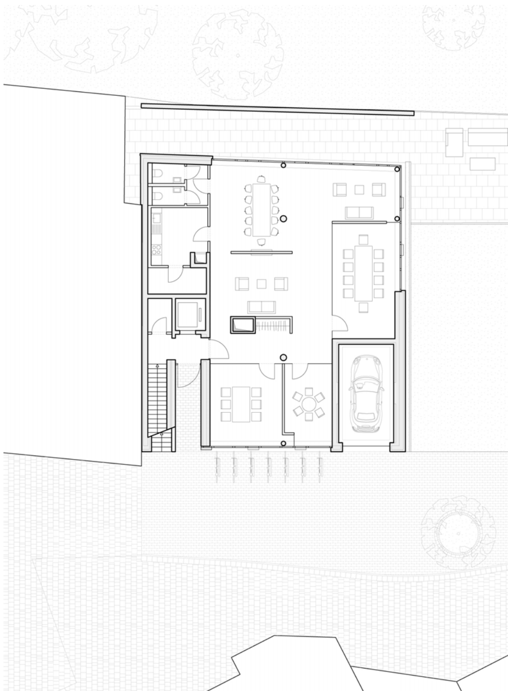
GRUNDRISSE EG, 1. OG M 1:200
