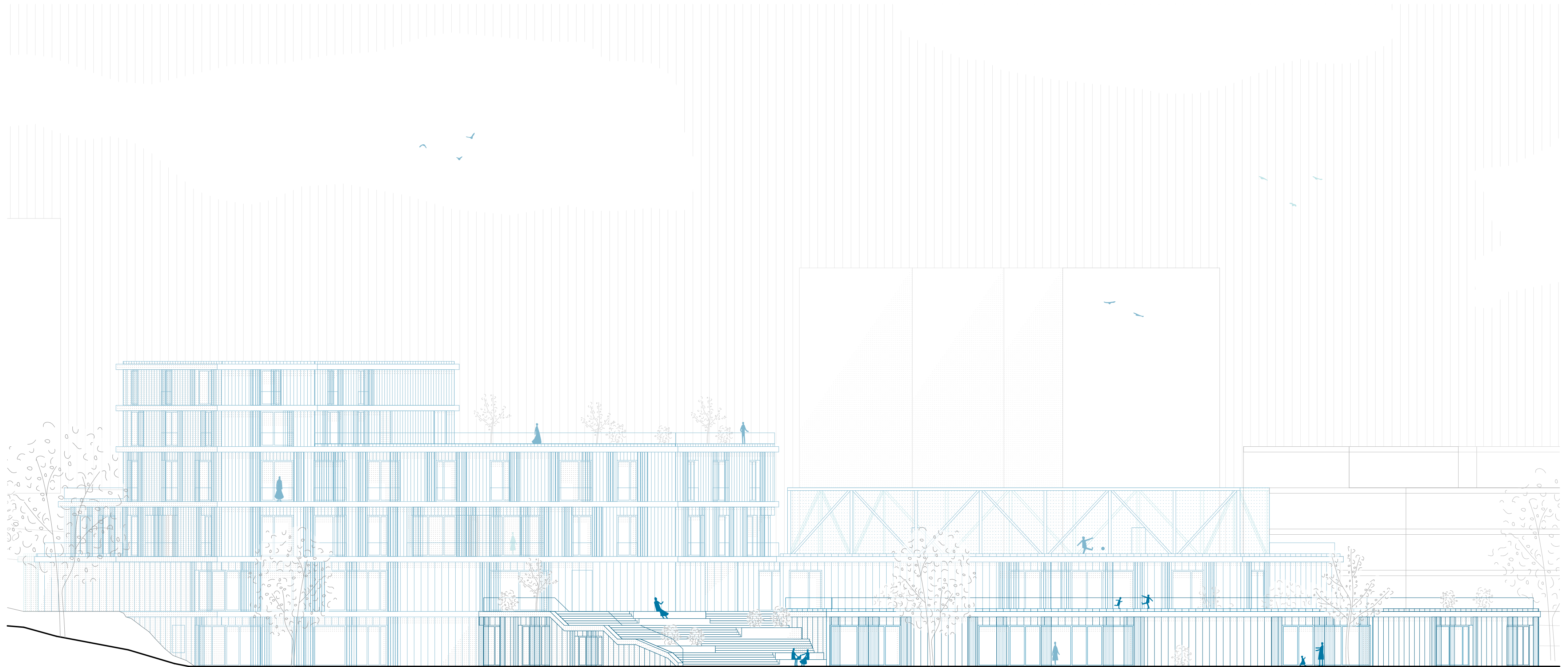
Ansicht Süd M 1:200
