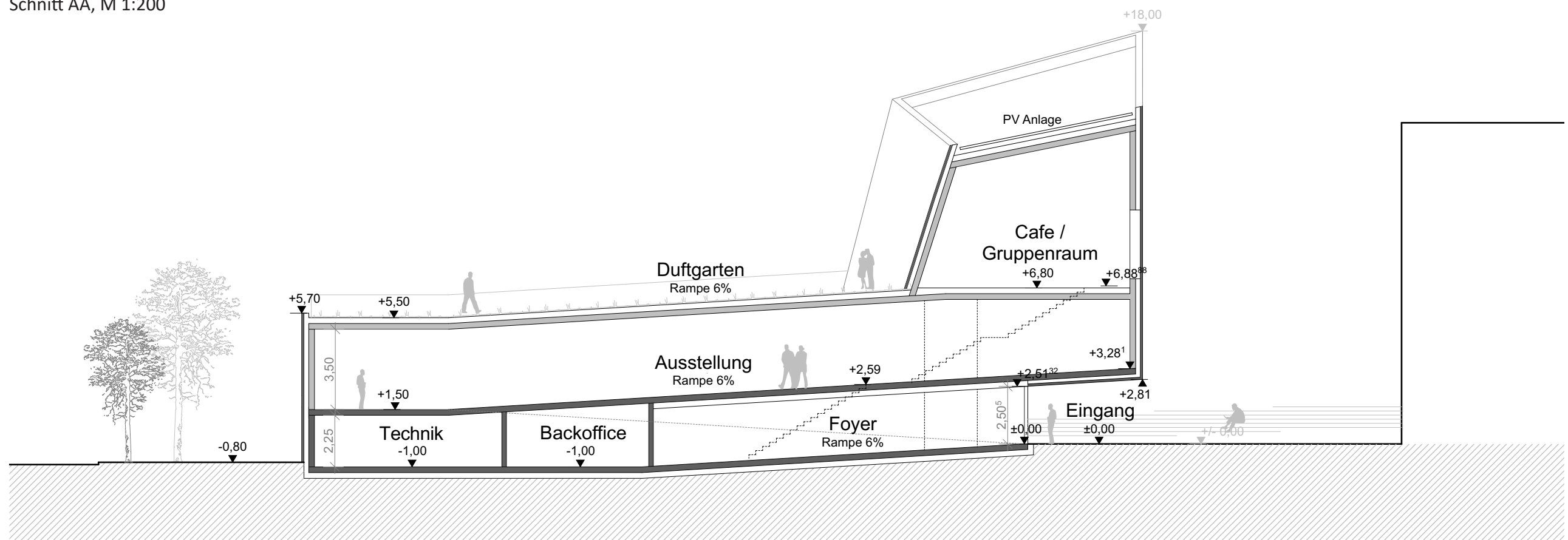
Schnitt BB, M 1:200
