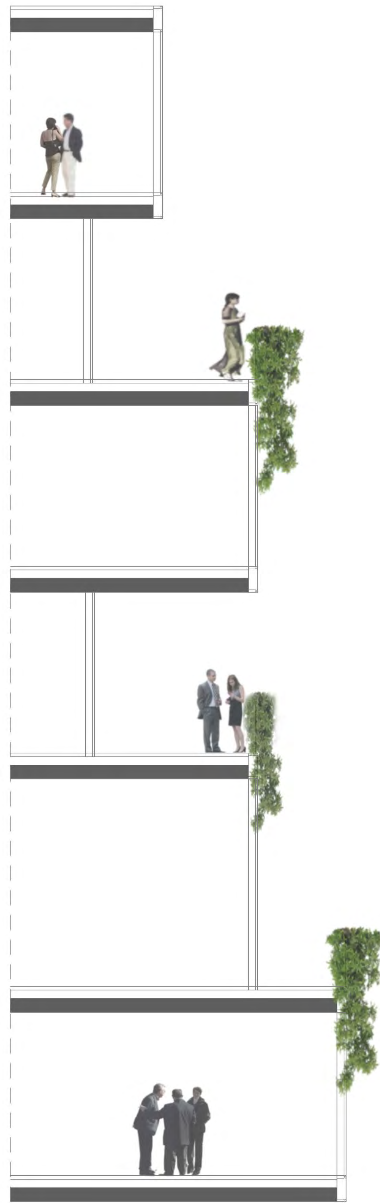
FASSADENSCHNITT M 1:50
