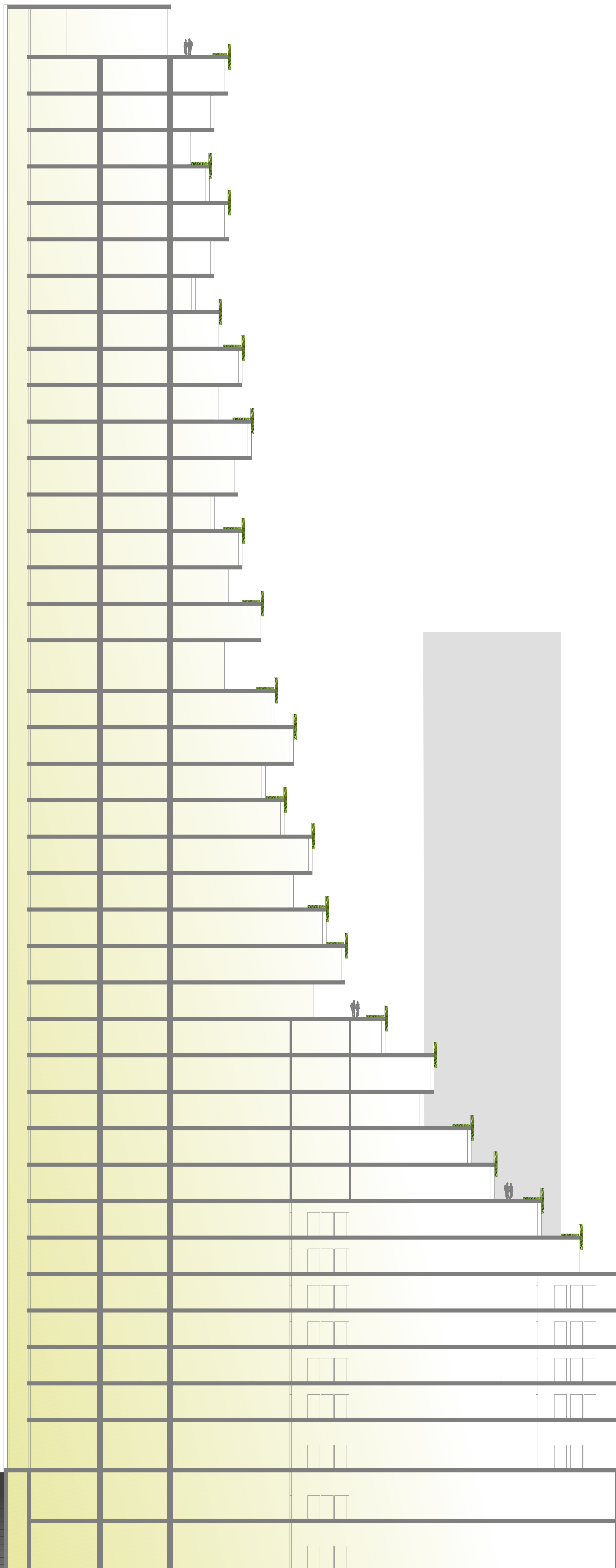
FASSADENSCHNITT M 1:50
