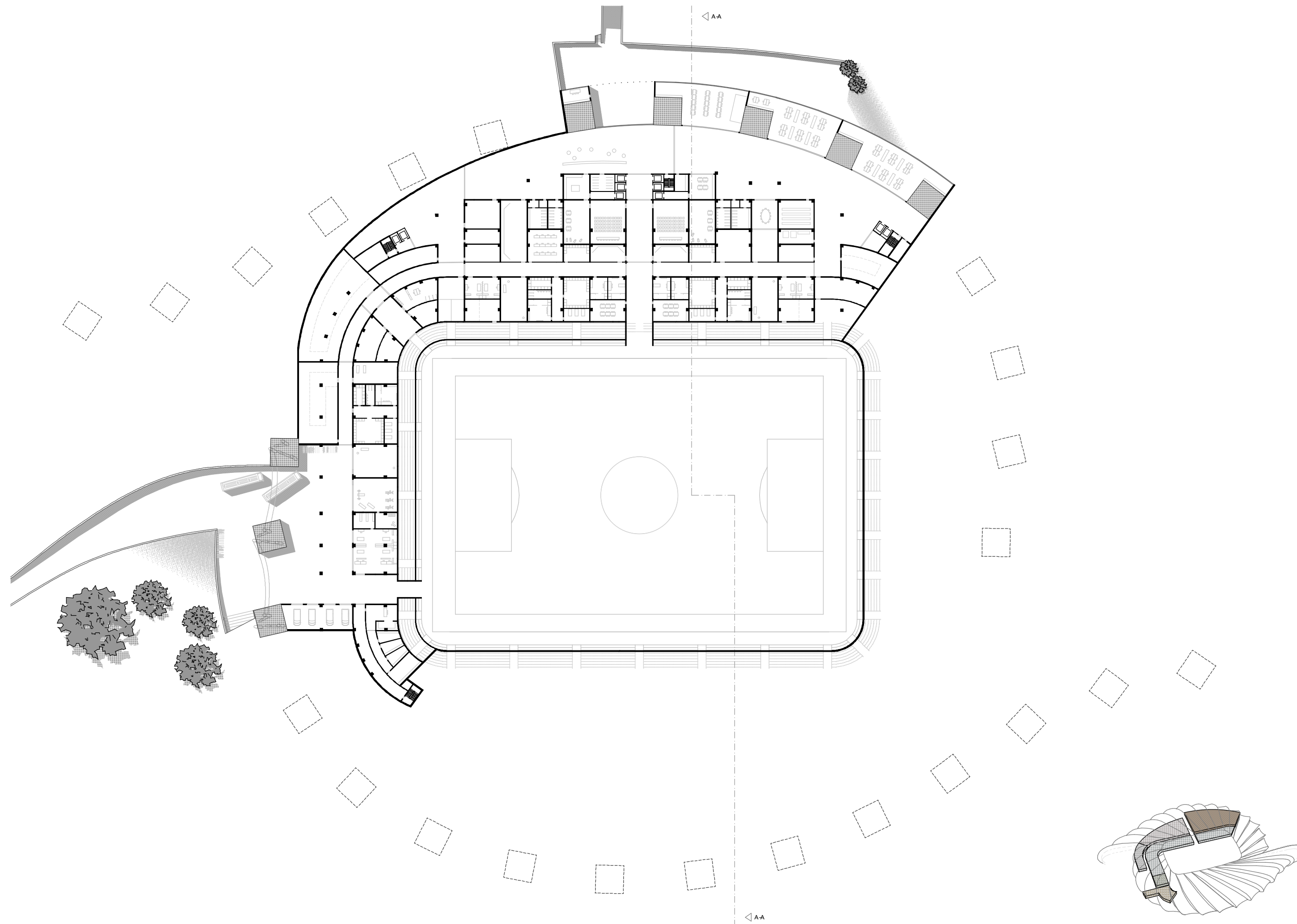
GRUNDRISS EBENE -1 1:1000
