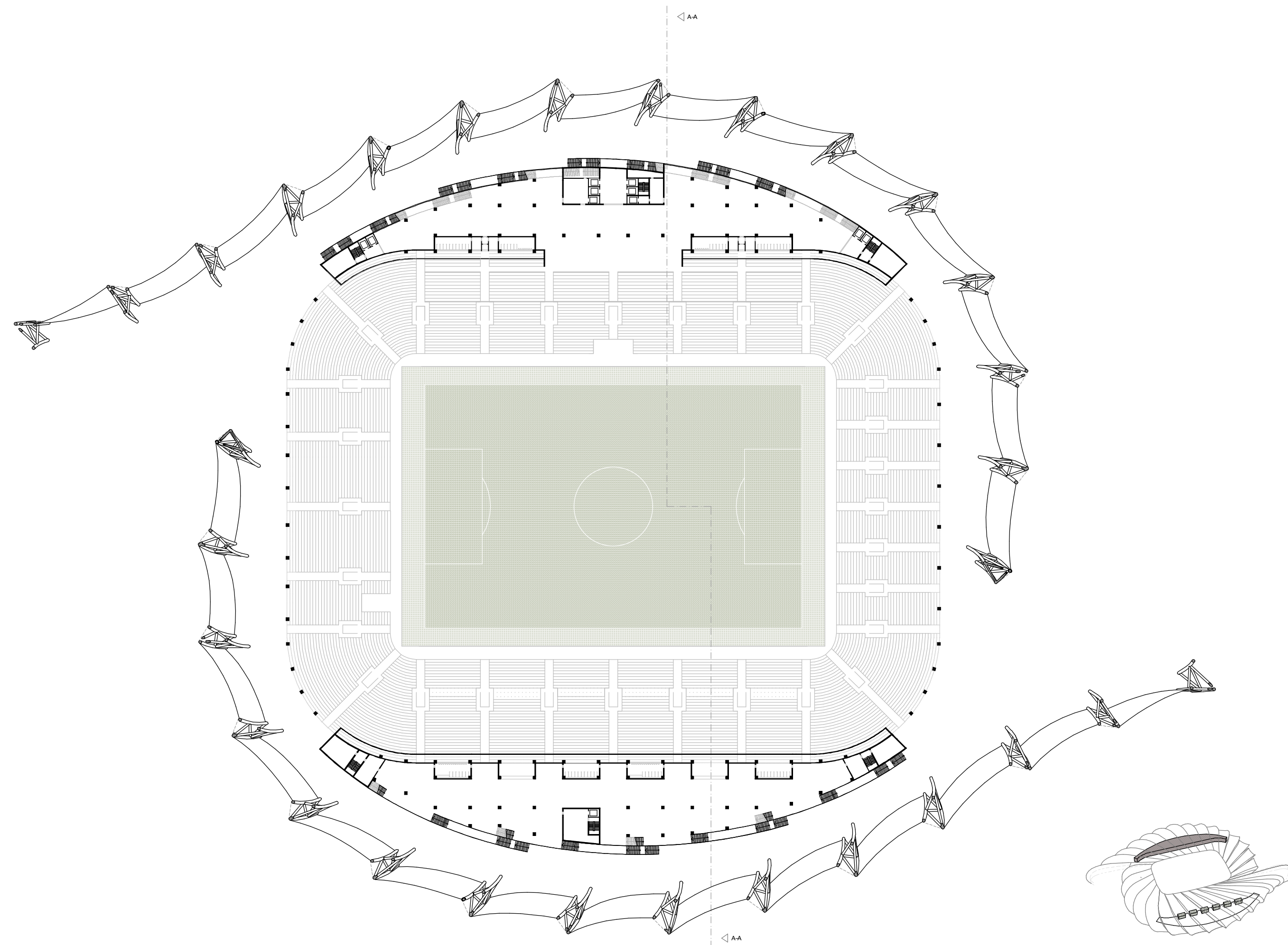
GRUNDRISS EBENE 1 1:1000
