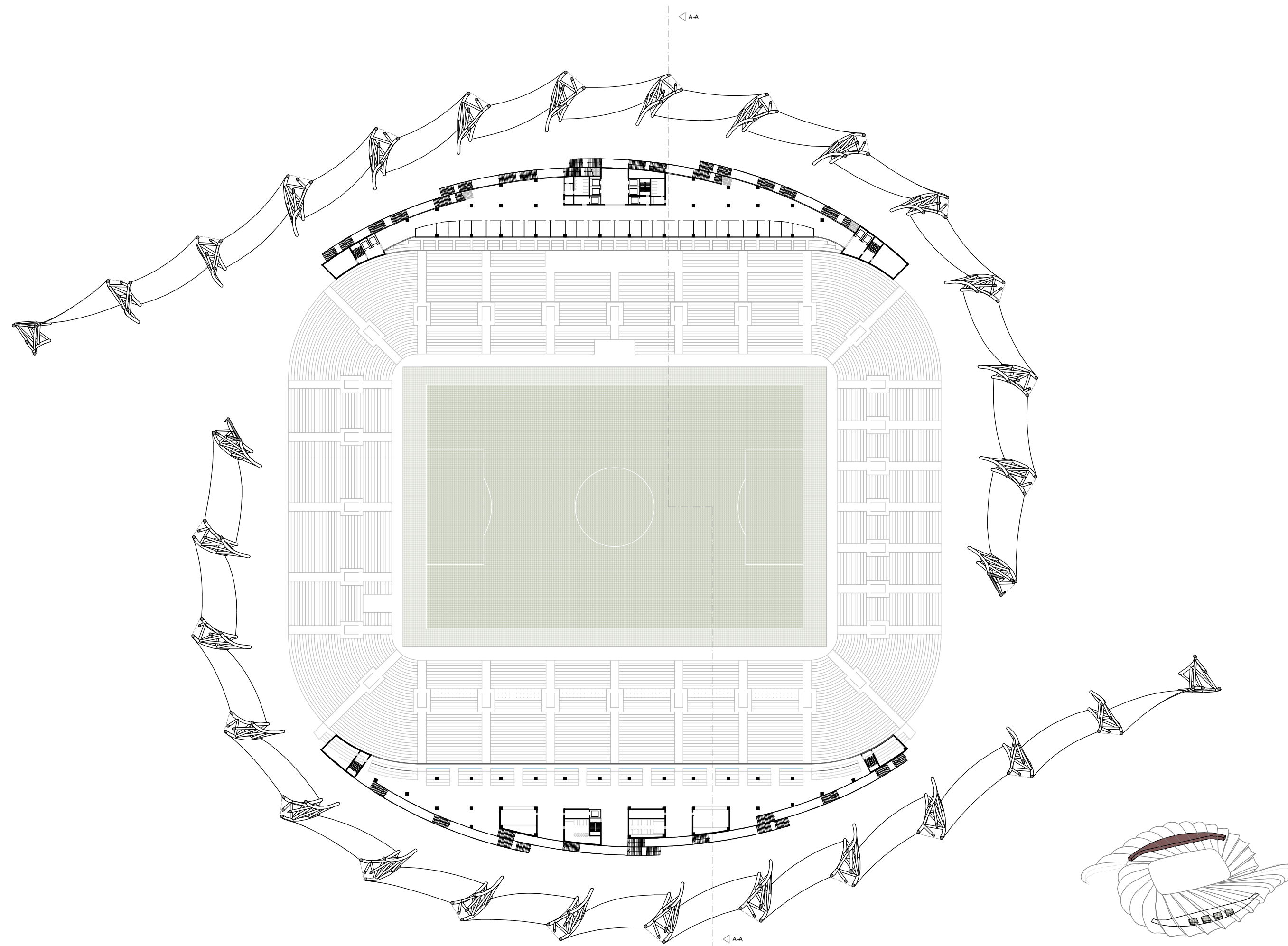
GRUNDRISS EBENE 2 1:1000
