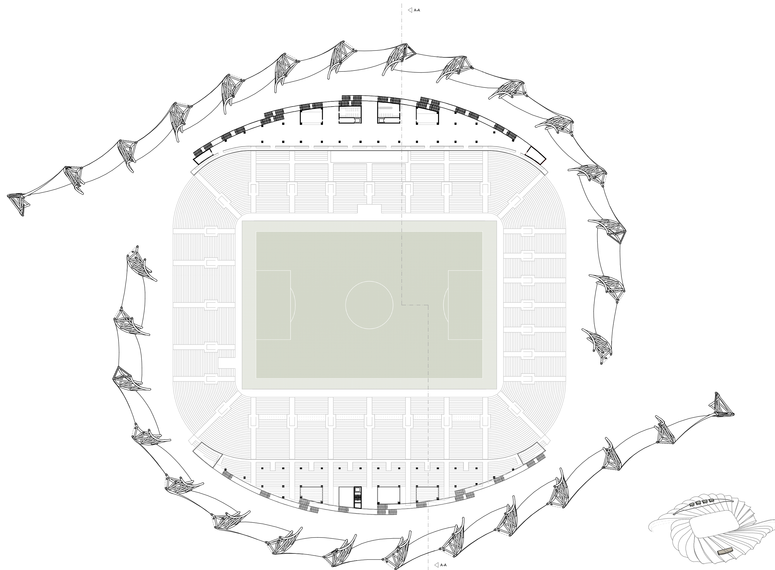
GRUNDRISS EBENE 3 1:1000
