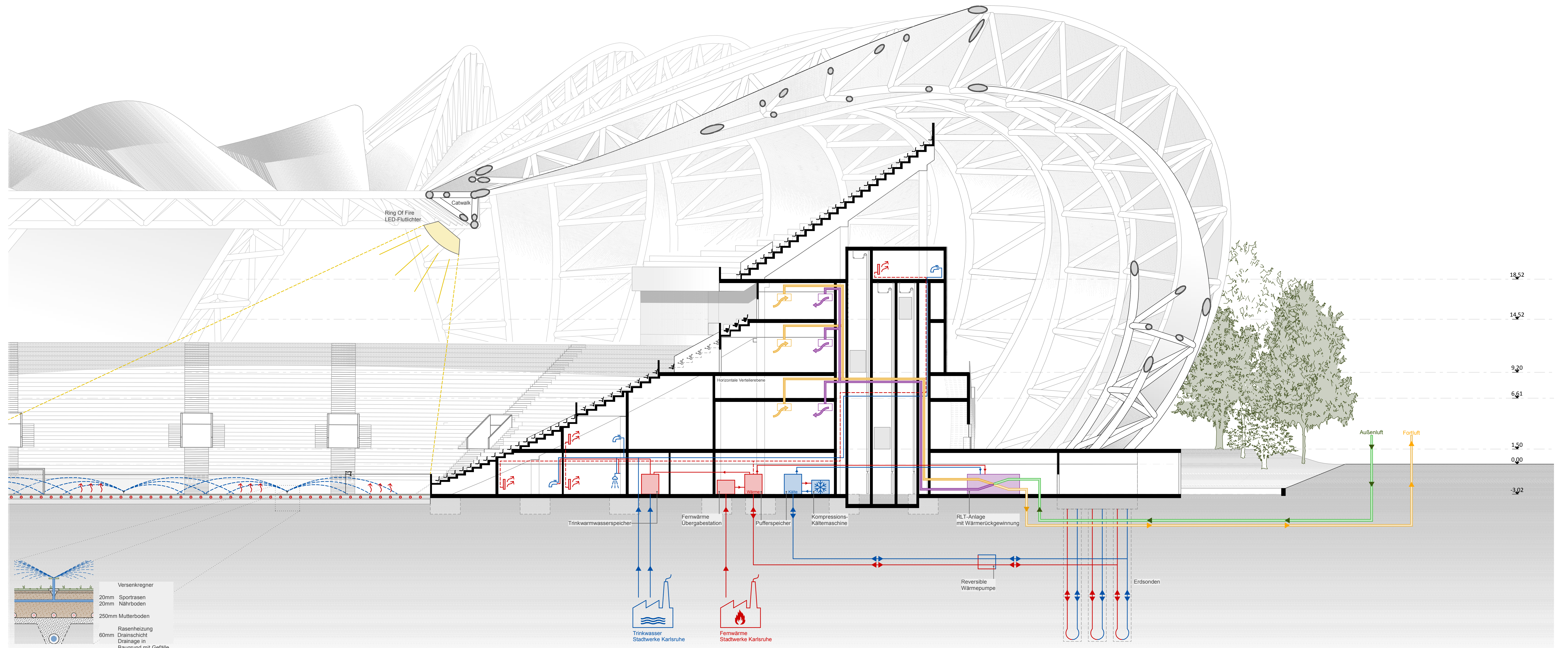
ENERGIE SCHNITT A-A 1:200
