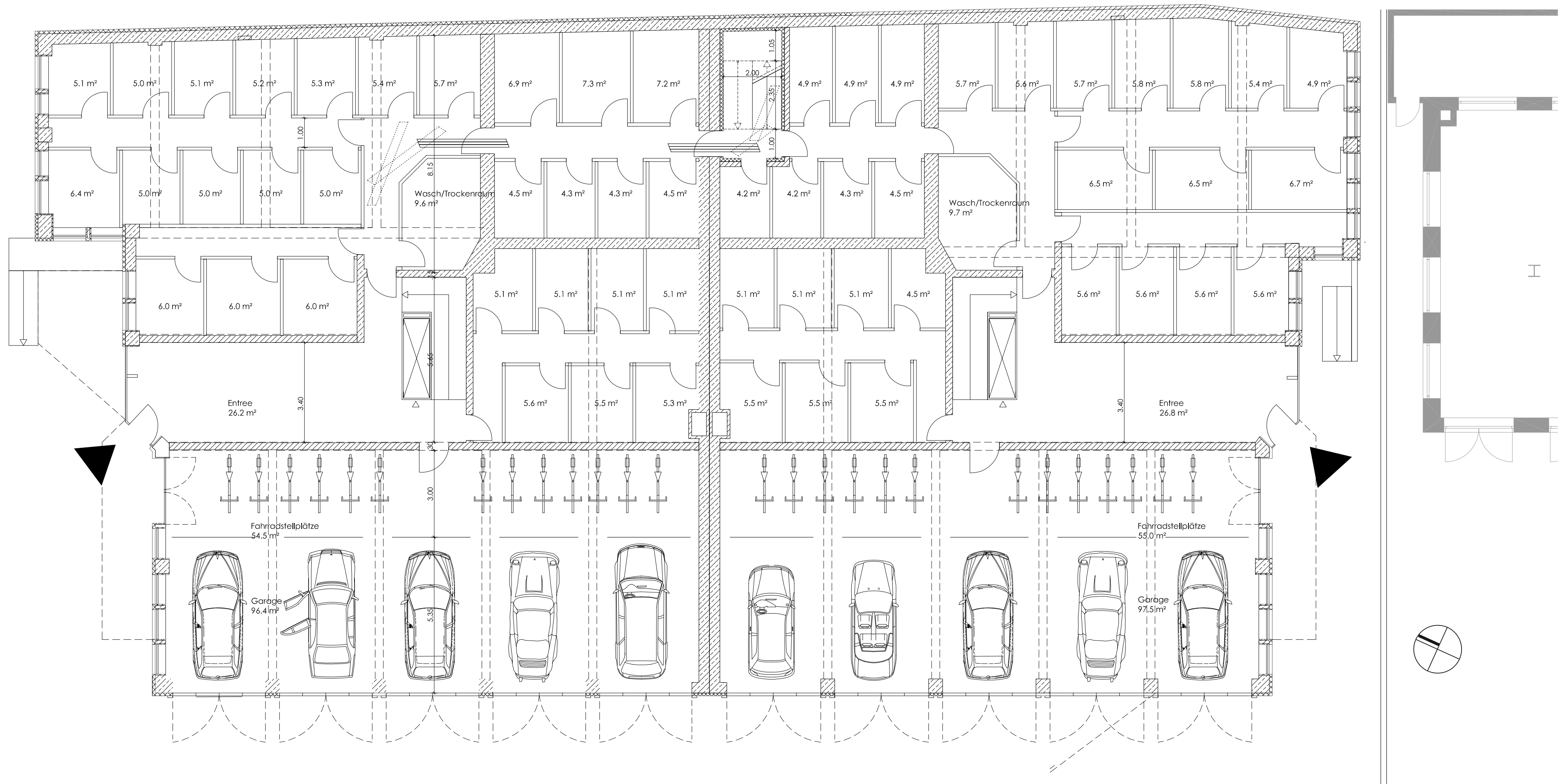
erdgeschoss m 1:100
