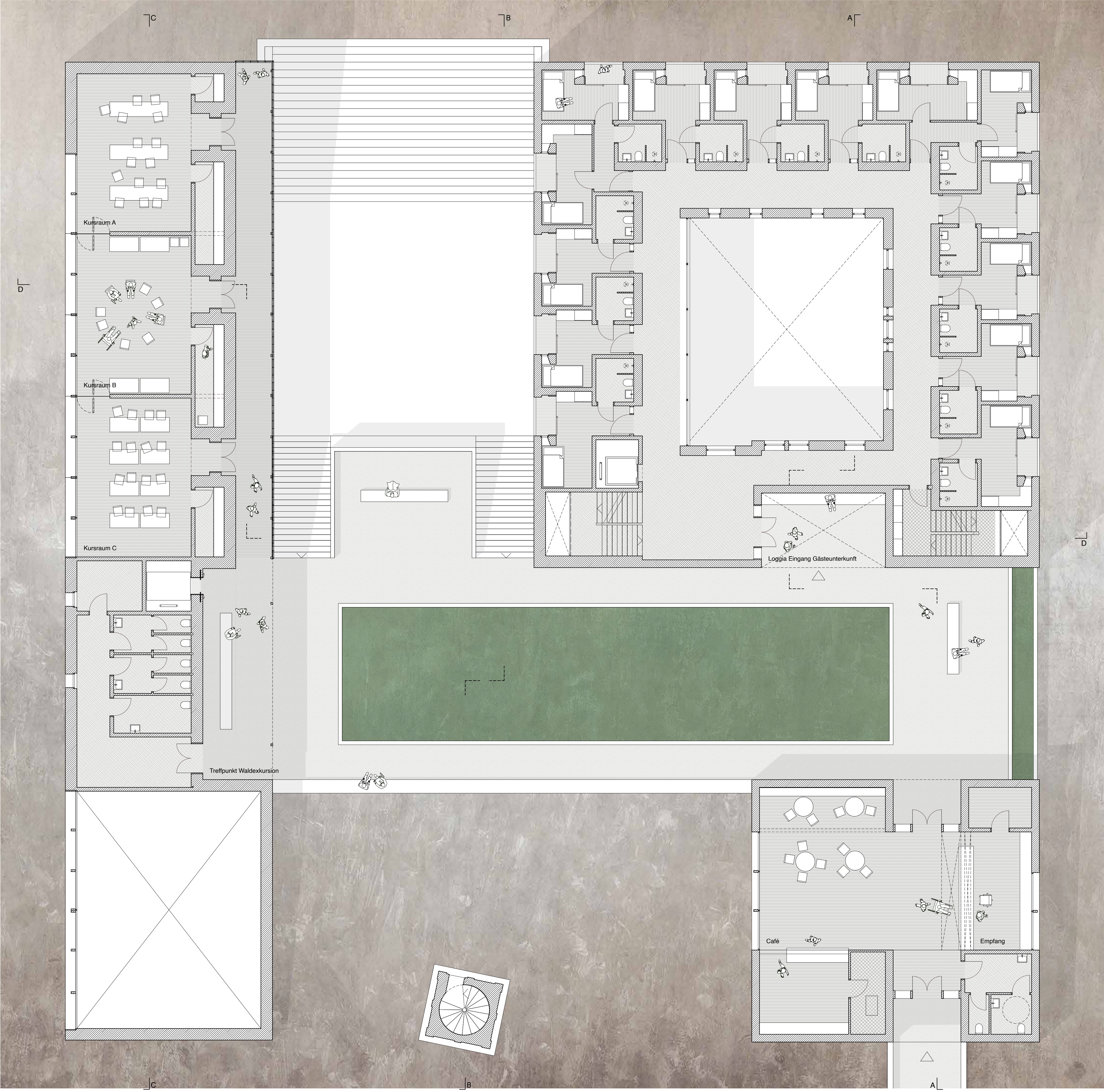
Grundriss Obergeschoss 1.100 Therapiezentrum - Königsberg Winter 19/20 Johanna Spies Maximilian Goetze
